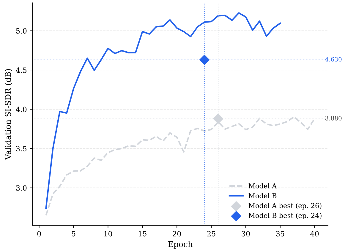
Validation SI-SDR per Epoch
