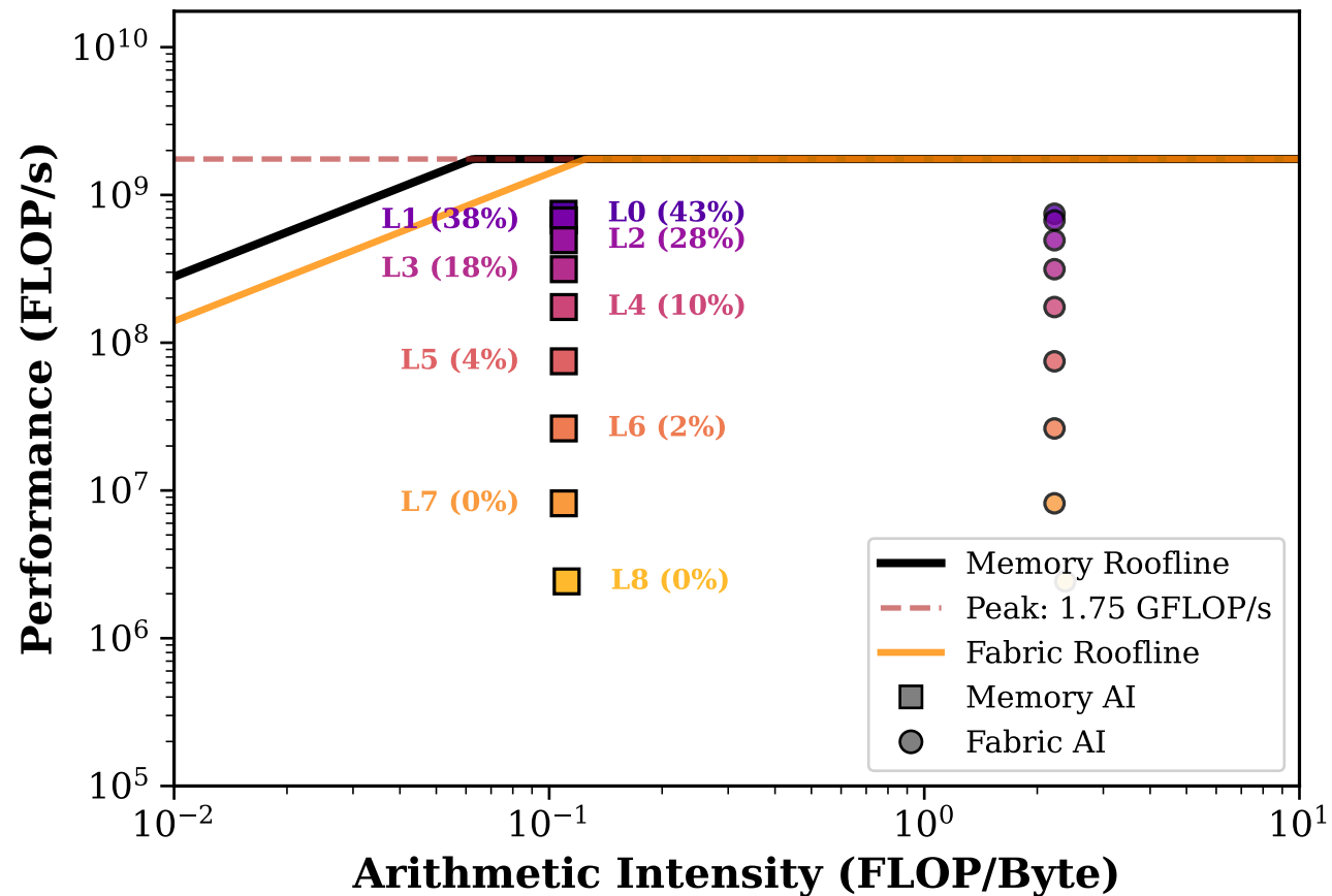
(a) Per PE(0,0)
