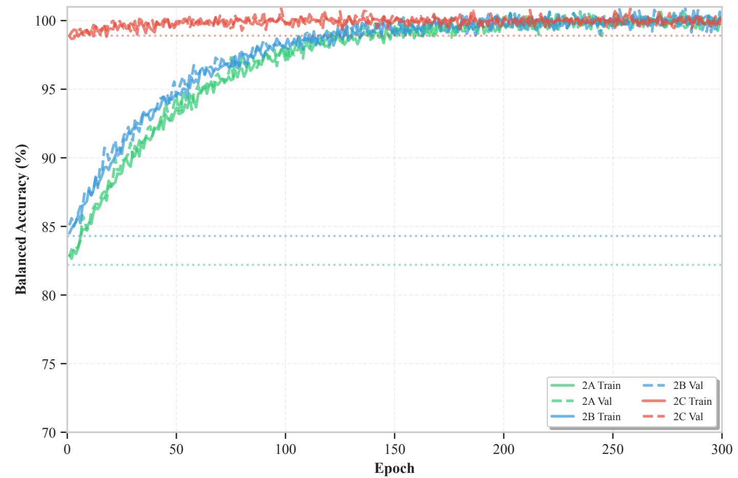
(d) Stage 2: Accuracy Convergence
