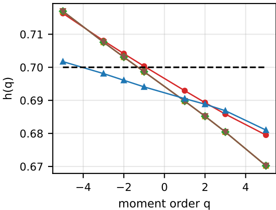
(a) fGn, H = 0.7
