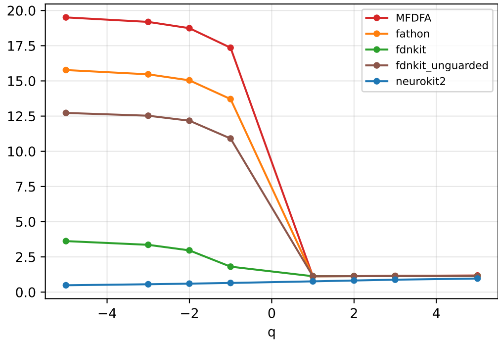
real EEG channel eegbci_s1_r4_Fc5
