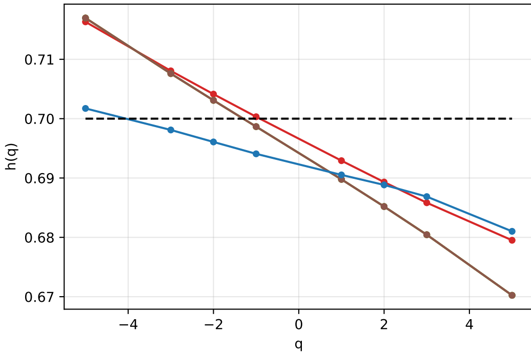
synthetic control, true h(q) = 0.7 fgn_H0.7
