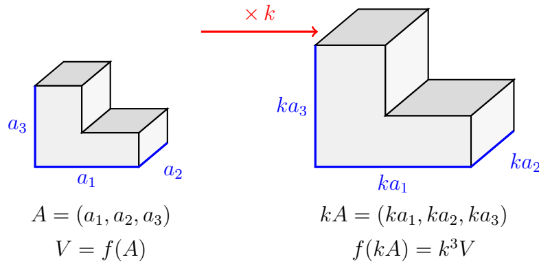
Рис. 4: Тело задано тройкой линейных размеров A = (a_1, a_2, a_3) , и объём мы считаем функцией этой тройки: V = f(A) . Преобразование масштаба умножает все три размера на одно и то же k : форма остаётся прежней, а объём вырастает в k^3 раз.
