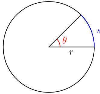
Рис. 1: Вот отсюда берутся радианы
