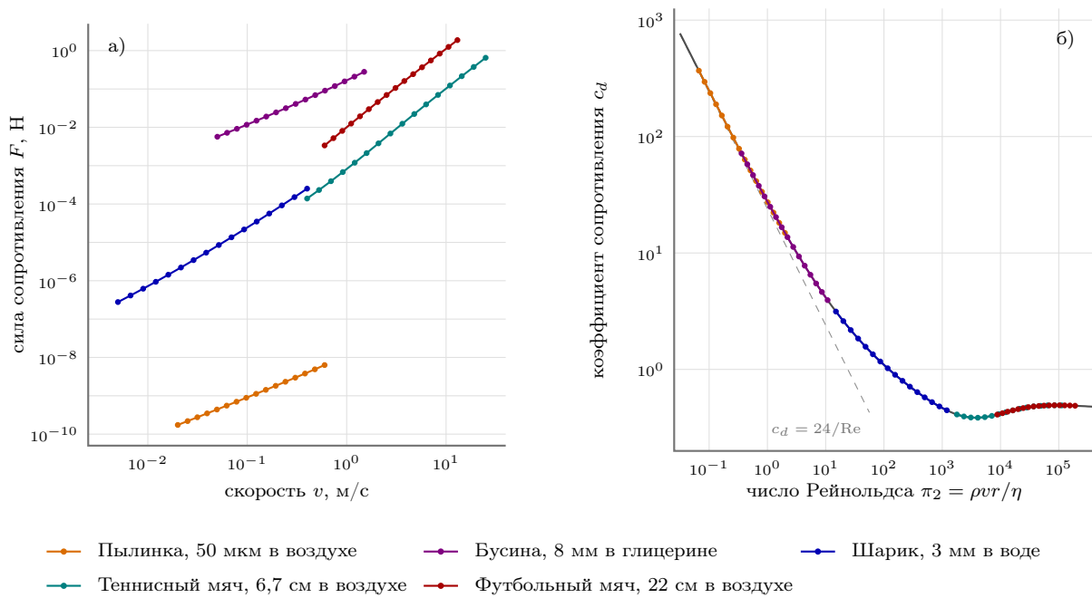
Рис. 5: Слева сила сопротивления против скорости для пяти тел: между крайними кривыми девять порядков по силе, и никакого общего закона в этих осях не видно. Справа те же самые числа в безразмерных осях: по горизонтали число Рейнольдса \pi_2 = \rho v r / \eta , по вертикали коэффициент сопротивления c_d = F / (\rho v^2 S / 2) , где S — площадь сечения тела; c_d есть \pi_1 / \pi_2 с точностью до числового множителя. Пять кривых садятся на одну, и это и есть зависимость \pi_1 = f(\pi_2) . Штриховая прямая — предел Стокса c_d = 24 / \text{Re} , к которому кривая выходит при малых числах Рейнольдса. Точки не измерены: они посчитаны по сводной кривой сопротивления шара (корреляция Клифта и Говена, 1971, описывающая усреднение семнадцати опытных работ) для пяти конкретных тел.
