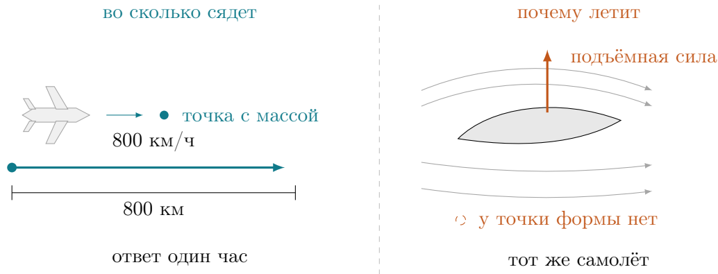
Рис. 6: Границу модели назначает вопрос, а не тело. Слева спрашивают, во сколько машина сядет, и она сжимается в точку. В ответ входят только путь и скорость, размах крыла в него не вошёл. Справа спрашивают, почему она летит, и точка не годится совсем, потому что подъёмную силу рождает форма крыла.
