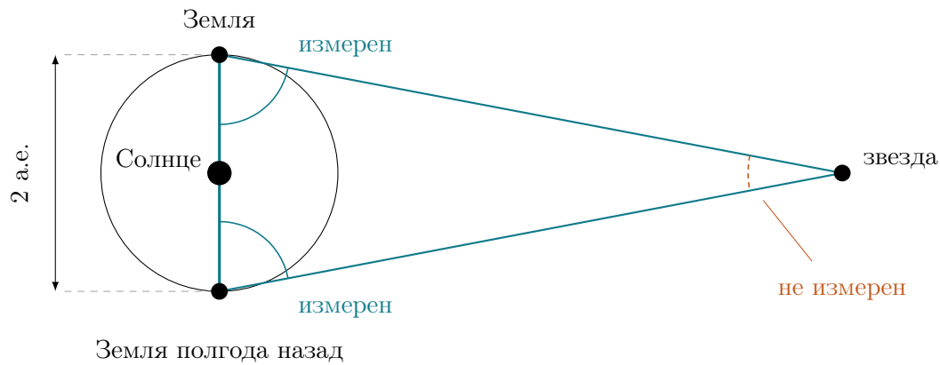
Рис. 4: Основание треугольника есть диаметр земной орбиты, две астрономические единицы, и с двух его концов звезда видна под чуть разными углами. Два угла при Земле измеряют, а третий, при звезде, не измеряет никто, и его получают в предположении, что геометрия плоская. Расстояние до звезды здесь не в масштабе, иначе звезда ушла бы далеко за поля.
