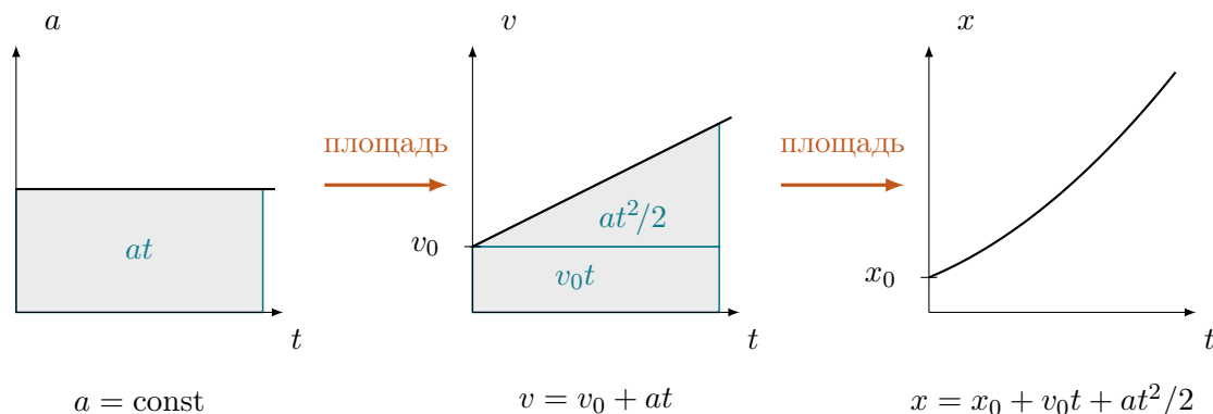
Рис. 18: Каждый график получается из предыдущего одним действием, площадью. Под горизонтальной прямой a(t) лежит прямоугольник, и площадь растёт как t . Под наклонной v(t) к прямоугольнику прибавляется треугольник, и площадь растёт как t^2 . Отсюда и разница между t в одной формуле и t^2 в другой.
