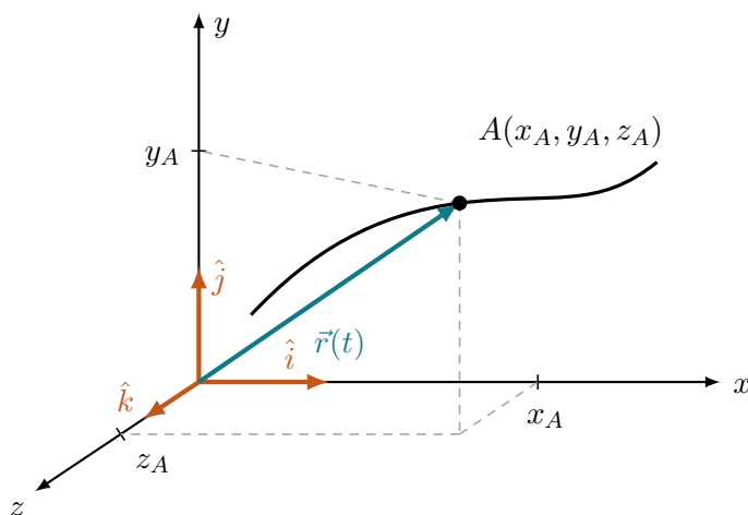
Рис. 10: Траектория движения материальной точки с радиус-вектором. Стрелка \vec{r}(t) соединяет начало координат с положением точки A(x_A, y_A, z_A) , а кривая показывает линию, по которой прошла точка. Штриховые линии — проекции точки на координатные оси.
