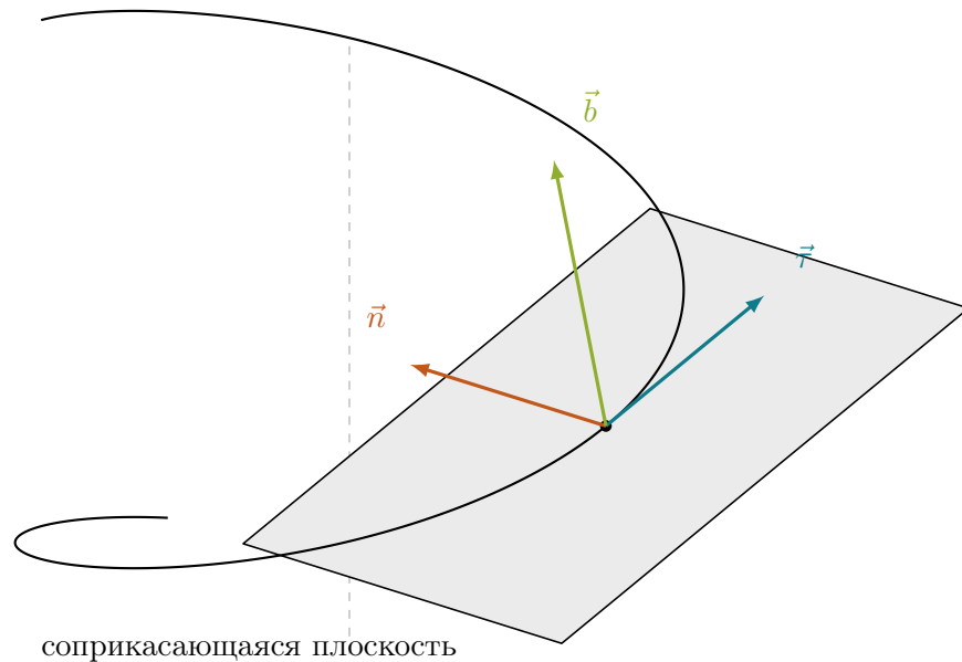
Рис. 27: На винтовой линии касательный вектор \vec{\tau} и нормаль \vec{n} натягивают соприкасающуюся плоскость, а бинормаль \vec{b} выходит из неё. Вдоль \vec{b} составляющей ускорения нет при любом движении, и третья ось нужна только для полноты тройки.
