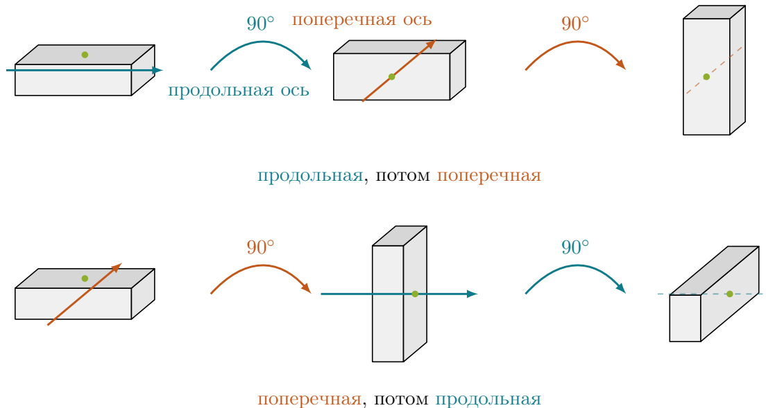
Рис. 23: Кирпич поворачивают на 90^\circ вокруг двух осей. В верхнем ряду сначала вокруг продольной, потом вокруг поперечной; в нижнем те же два поворота в обратном порядке. Отмеченная точка приходит в разные места, и конечные положения кирпича разные. Конечные повороты не перестановочны, поэтому вектором они не складываются.
