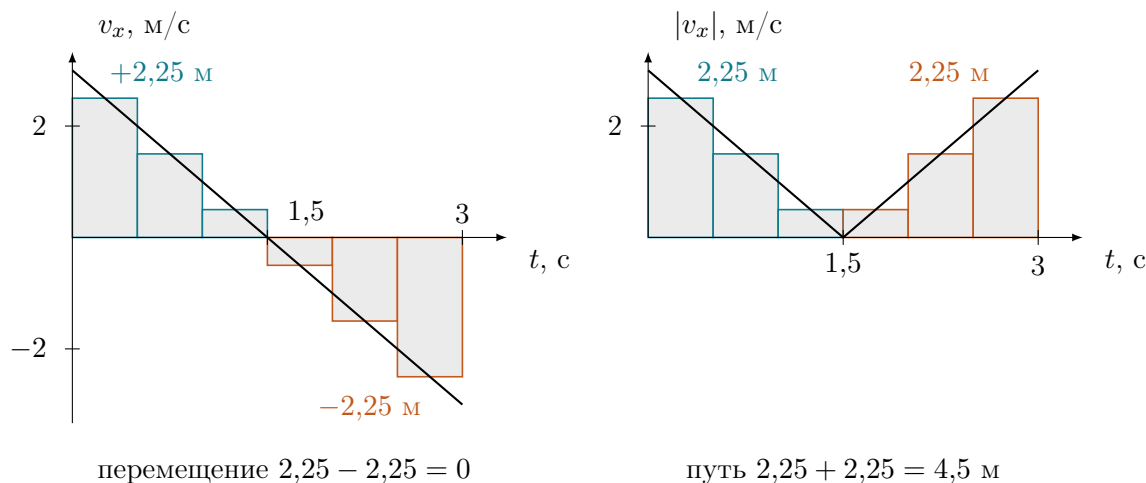
Рис. 17: Слева проекция скорости v_x = 3 - 2t меняет знак, столбики уходят под ось и входят в перемещение со знаком минус: за три секунды точка набирает 2,25 м вперёд и столько же теряет, перемещение равно нулю. Справа те же столбики сложены по модулю и дают путь 4,5 м.
