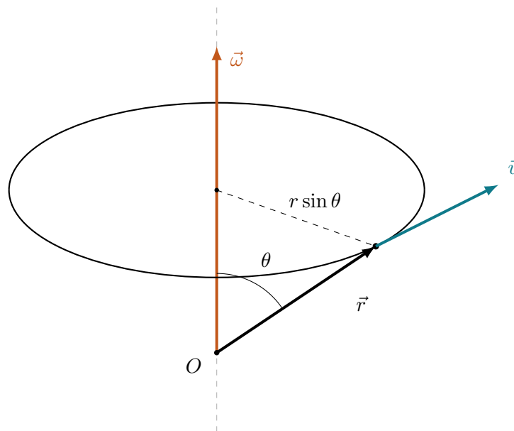
Рис. 22: Угловая скорость \vec{\omega} направлена вдоль оси вращения, радиус-вектор \vec{r} проведён из начала к точке, а угол между ними обозначен \theta . Точка ходит по окружности радиуса r \sin \theta , то есть по расстоянию до оси, а не до начала. Линейная скорость \vec{v} = \vec{\omega} \times \vec{r} лежит по касательной к этой окружности, и её направление даёт правило правой руки.
