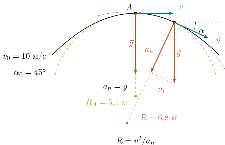
Рис. 29: В вершине скорость горизонтальна, всё ускорение поперечно, и радиус кривизны равен 5,1 м. В наклонной точке \vec{g} разложен вдоль скорости и поперёк неё, поперечная составляющая меньше, и радиус вырастает до 6,8 м. Здесь два маршрута счёта кривизны сходятся в одной точке.
