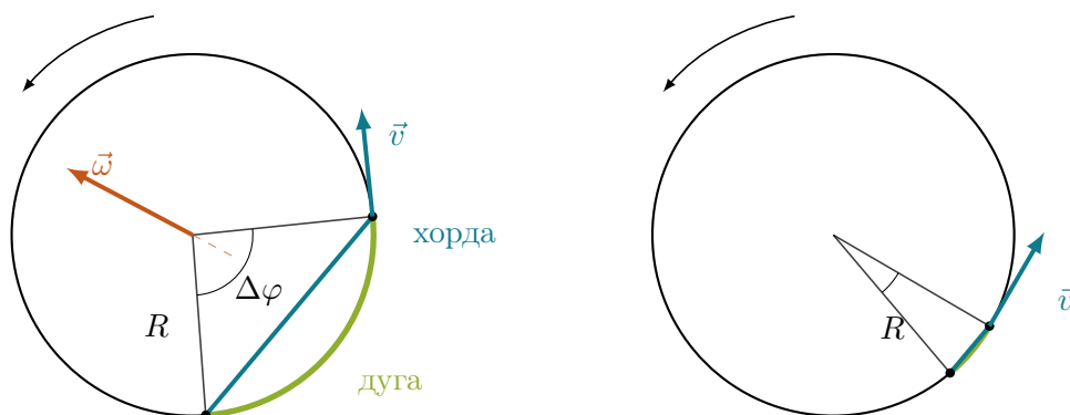
Рис. 21: На левой окружности угол \Delta\varphi взят большим, и хорда 2R \sin(\Delta\varphi/2) заметно короче дуги R\Delta\varphi . На правой тот же угол мал, и они сливаются. Отсюда и берётся связь v = \omega R , потому что в пределе отношение хорды к дуге стремится к единице.
