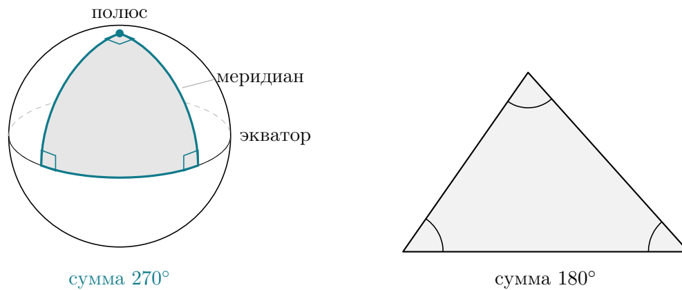
Рис. 2: Треугольник из четверти экватора и двух меридианов даёт сумму углов 270^\circ вместо 180^\circ , и все три его угла прямые. На проекции прямой угол прямым не выглядит, поэтому квадратики поставлены по касательным, посчитанным в трёх измерениях. Справа тот же вопрос на плоскости, где сумма равна 180^\circ .
