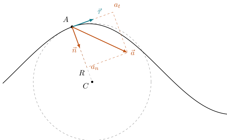
Рис. 26: На малом участке кривую заменяет окружность радиуса R с центром C , окружность кривизны, проведённая через три близкие точки кривой. В точке A касательный вектор \vec{\tau} ведёт вдоль траектории, нормаль \vec{n} смотрит на центр кривизны, и полное ускорение \vec{a} раскладывается по этой паре на тангенциальное a_t и нормальное a_n .
