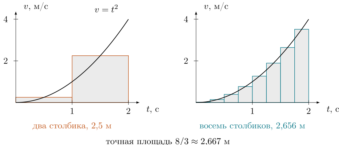
Рис. 16: Скорость v(t) = t^2 на промежутке от нуля до двух секунд. Два широких столбика дают 2,5 м, восемь узких дают 2,656 м, а точное значение интеграла равно 8/3 \approx 2,667 м. При каждом удвоении числа столбиков ошибка падает вчетверо.
