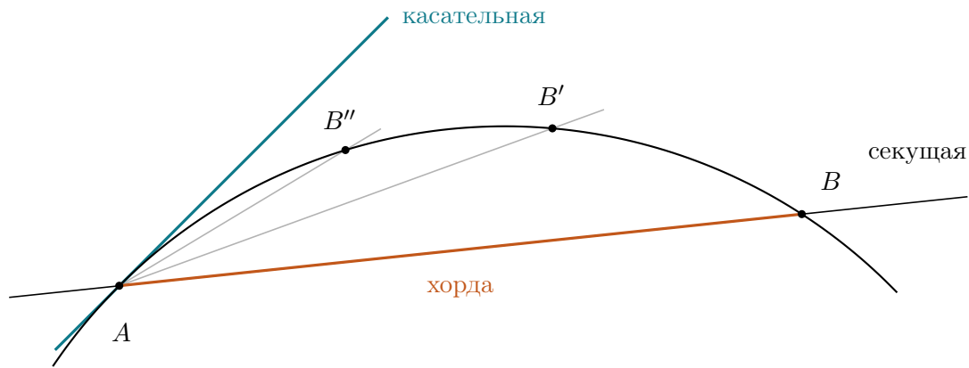
Рис. 13: Точка B пододвигается к A , хорда укорачивается, и секущая через две точки поворачивается, ложась на касательную в A . Направление отношения устанавливается, пока сама хорда исчезает: это и есть первый возврат языка.
