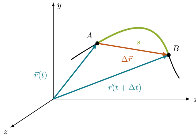
Рис. 12: Радиус-векторы для разных моментов времени и вектор перемещения. Здесь \vec{r}(t) и \vec{r}(t + \Delta t) задают положения A и B , а их разность \Delta\vec{r} соединяет эти точки хордой. Отдельным цветом показан путь s , длина самой дуги от A до B . На этом участке он в 1,2 раза длиннее хорды, а короче её не бывает никогда.
