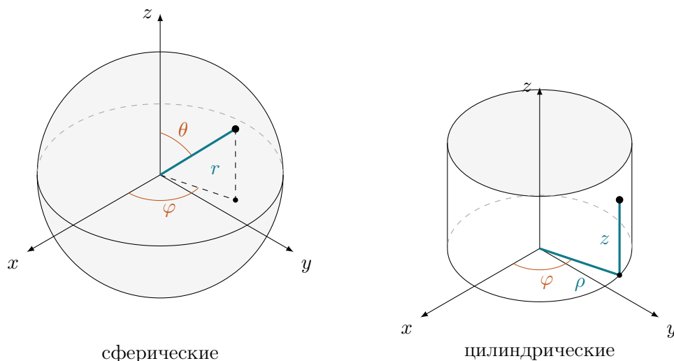
Рис. 8: Слева точка на сфере задана расстоянием r до начала, углом \theta от оси z и углом \varphi в плоскости xy . Справа та же точка задана расстоянием \rho до оси z , тем же углом \varphi и высотой z . Полярные координаты получаются из цилиндрических, если выбросить z .
