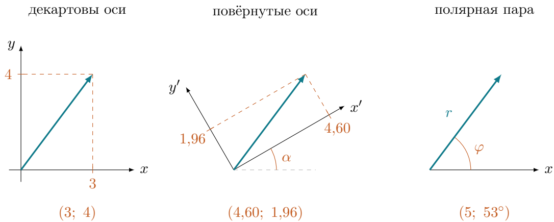
Рис. 7: Стрелка из начала в точку одна и та же во всех трёх случаях, а числа под ней разные. В декартовых осях это (3; 4) . В тех же осях, повёрнутых на 30^\circ , уже (4,60; 1,96) , а полярной парой (5; 53^\circ) . Столбик чисел наполовину наш, и это цена четвёртой договорённости.
