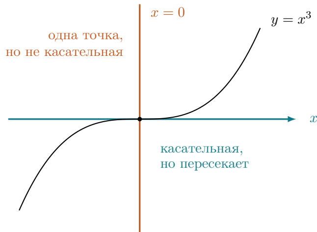
Рис. 14: Кривая y = x^3 разбивает школьное «касательная имеет с кривой одну общую точку» в обе стороны. Вертикальная прямая x = 0 имеет с кривой ровно одну общую точку и касательной не является. Ось x касательной является и при этом переходит с одной стороны кривой на другую.
