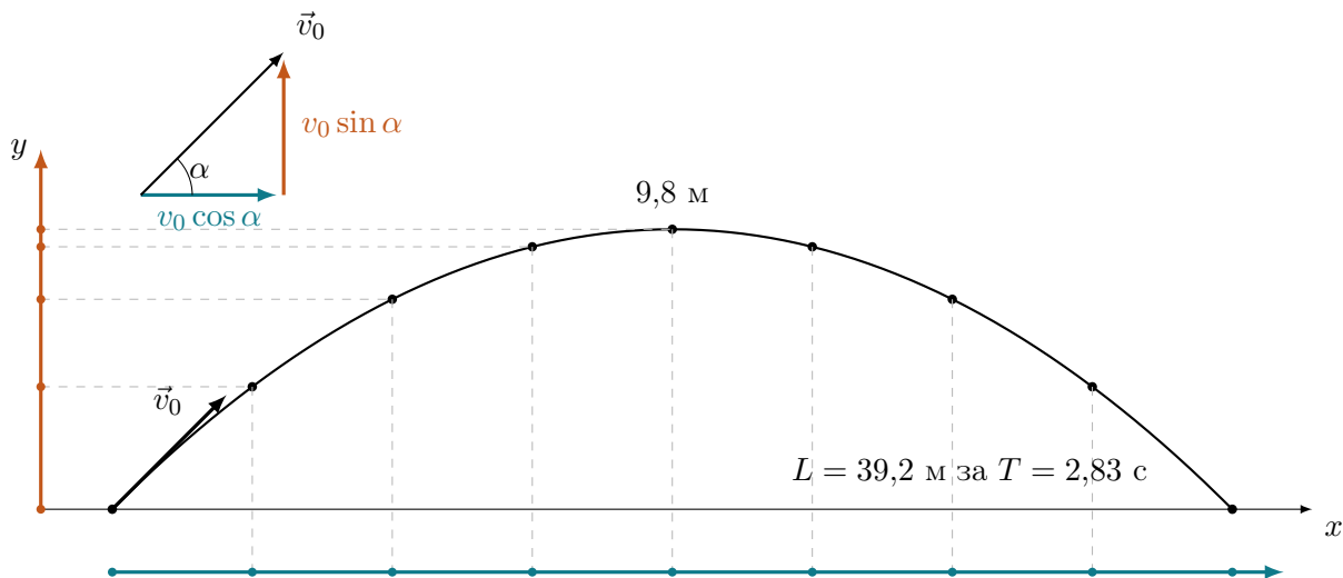
Рис. 19: Мяч отмечен в девяти положениях через равные промежутки времени. Вдоль горизонтали ускорения нет, эта строка столбца вырождается, и отметки внизу стоят на равных расстояниях. Вдоль вертикали ускорение -g работает целиком, и отметки слева сгущаются к вершине. Разница между t в одной формуле и t^2 в другой видна прямо по отметкам.
