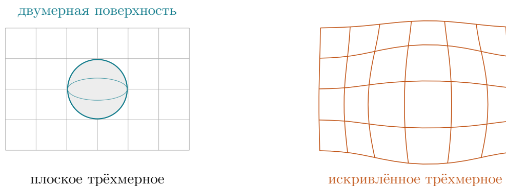
Рис. 3: Сфера есть двумерная поверхность внутри обычного плоского трёхмерного пространства, и её кривизну видно снаружи. Кривизна самого трёхмерного пространства такого взгляда со стороны не допускает, потому что выйти из него и поглядеть некуда. Решётка справа изогнута в самой себе, и прямых линий в ней не осталось. Оттого сфера соседнего рисунка работает картинкой, а не доказательством.
