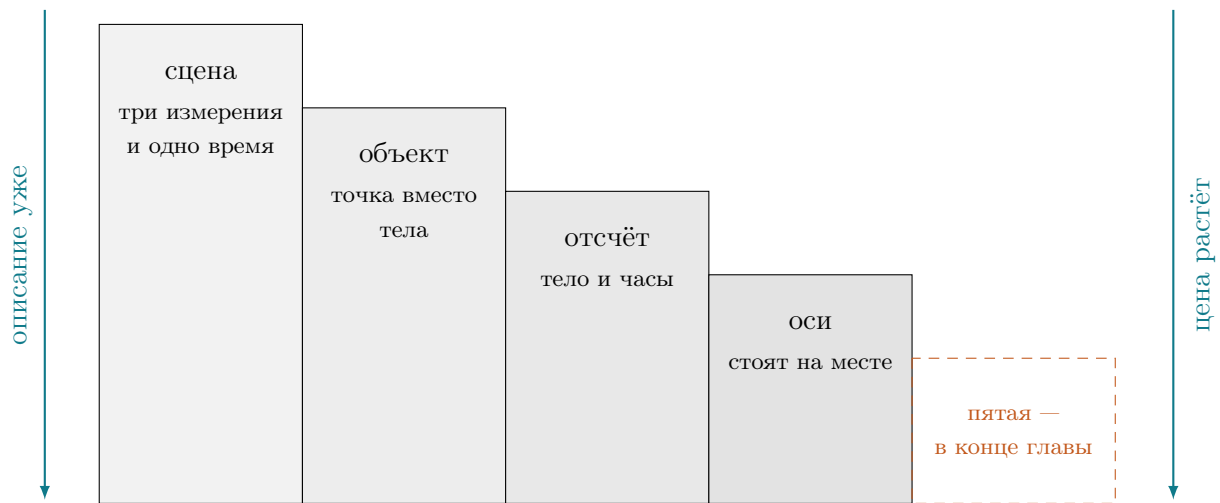
Рис. 1: Четыре договорённости берутся заранее, до всякой хитрой математики, и каждая сужает описание: сцена, объект, отсчёт, оси. Пятая стоит пустой, потому что собрать её раньше не из чего; её место в конце главы, в разделе о нормальном и тангенциальном ускорении. Чем ниже ступень, тем уже описание и тем дороже за неё плачено.
