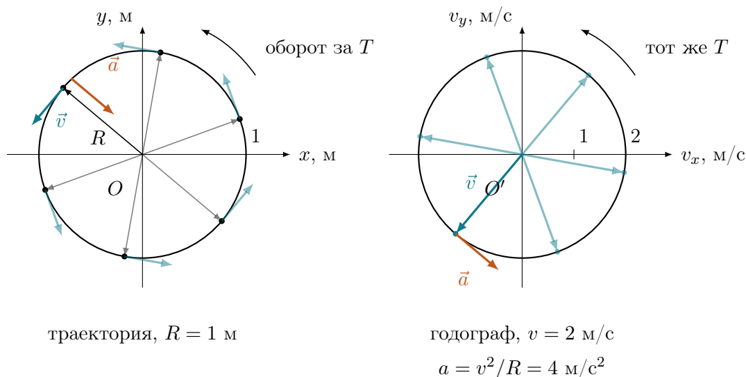
Рис. 20: Слева траектория радиуса R с центром O , точка в шести положениях через равные углы, и в каждом скорость по касательной; все стрелки одной длины, потому что движение равномерное. Справа те же стрелки отложены из общего начала O' , и их концы легли на окружность радиуса v . У выделенной пары справа показано ускорение по касательной к годографу, слева тот же вектор перенесён в точку и смотрит в центр.
