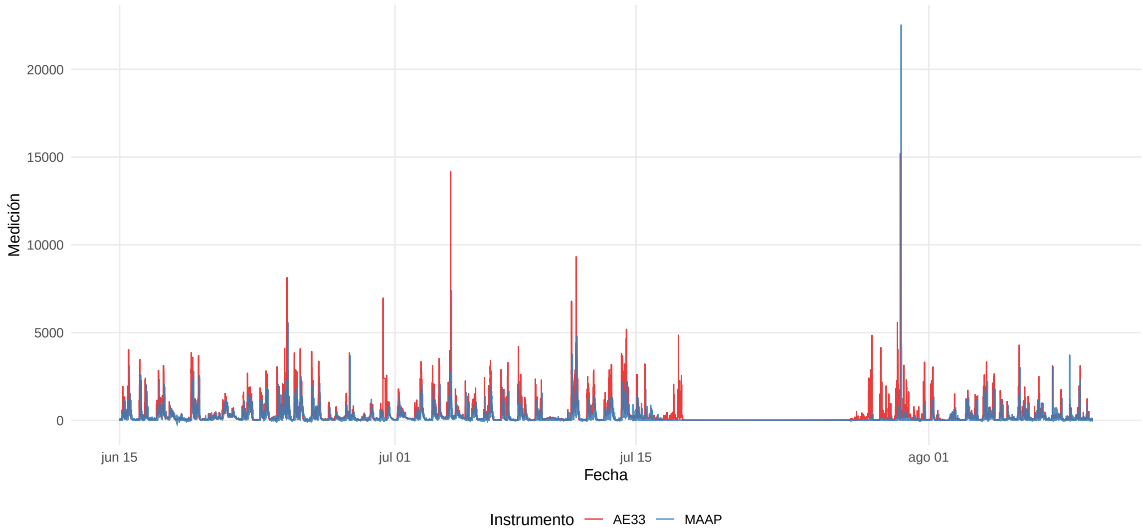
Series temporales: AE33 y MAAP
