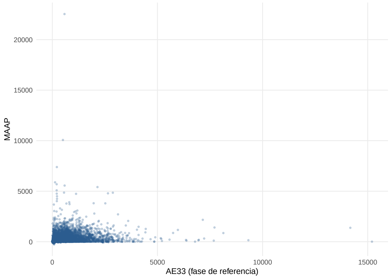
Nube de puntos: AE33 (fase de referencia) vs MAAP
