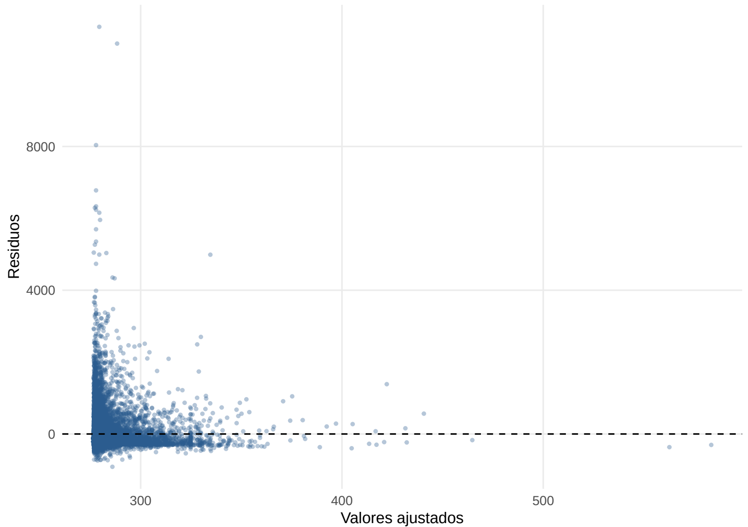
Residuos de regresión: AE33 (solapamiento) vs AE36 (solapamiento)
