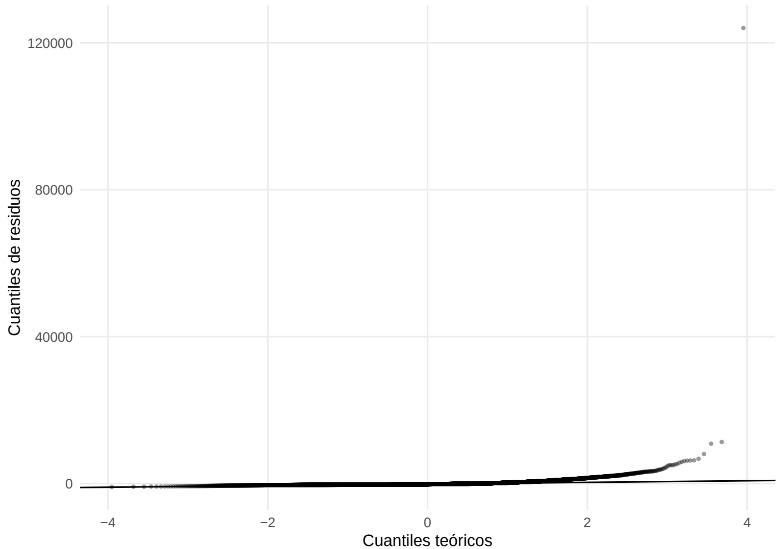
QQ-plot de residuos: AE33 crudo vs AE36 crudo
