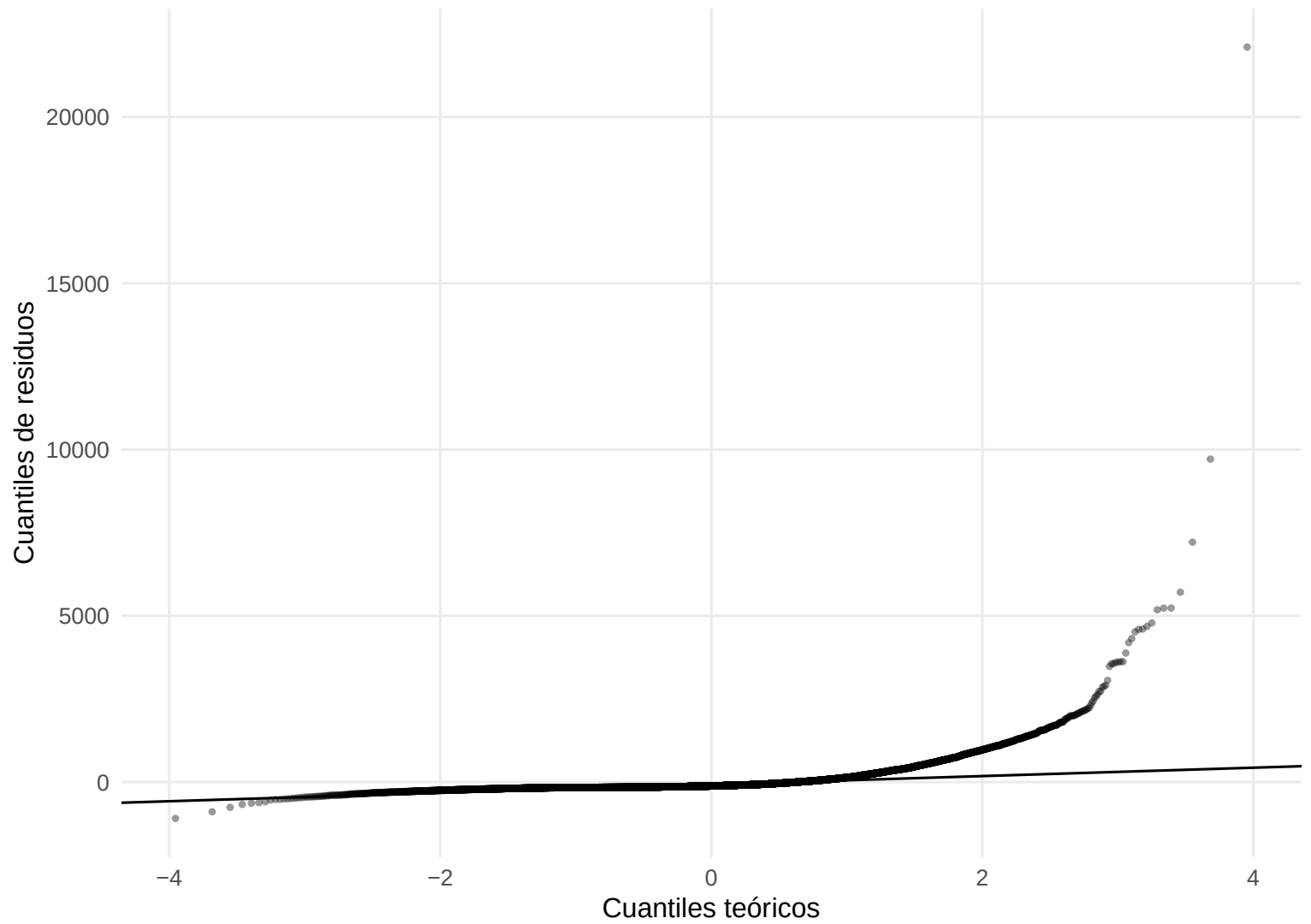
QQ-plot de residuos: AE36 vs MAAP
