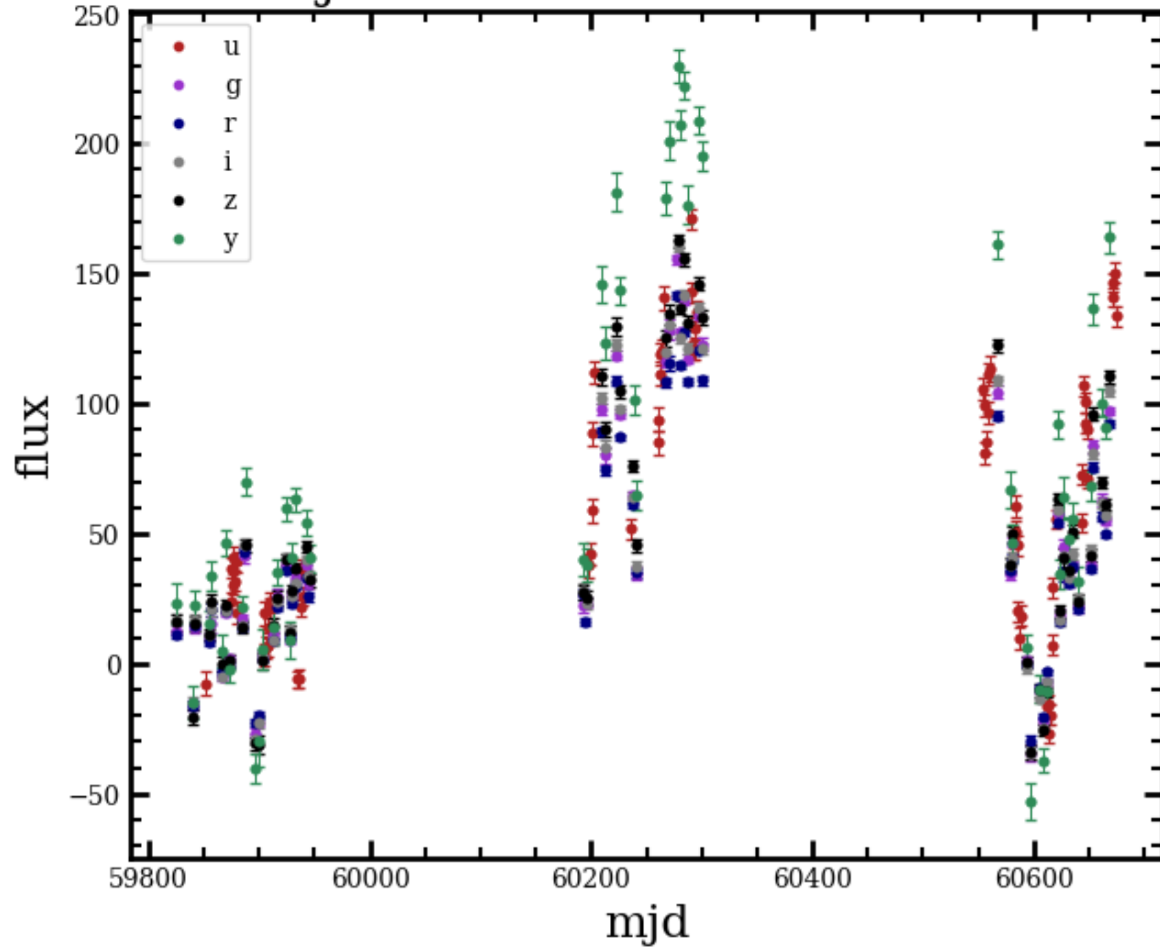
object ID: 71676 -- class: AGN
