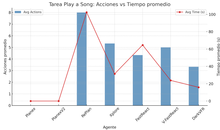
Figure 7.3: Rendimiento de los agentes (N. Acciones vs Tiempo promedio) en el entorno Play a Song . Fuente: Elaboración propia.
