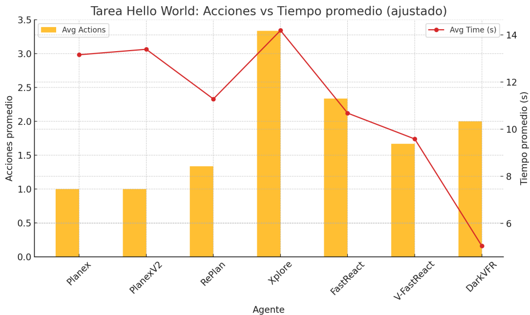
Figure 7.1: Rendimiento de los agentes (N. Acciones vs Tiempo promedio) en el entorno Hello World . Fuente: Elaboración propia.
