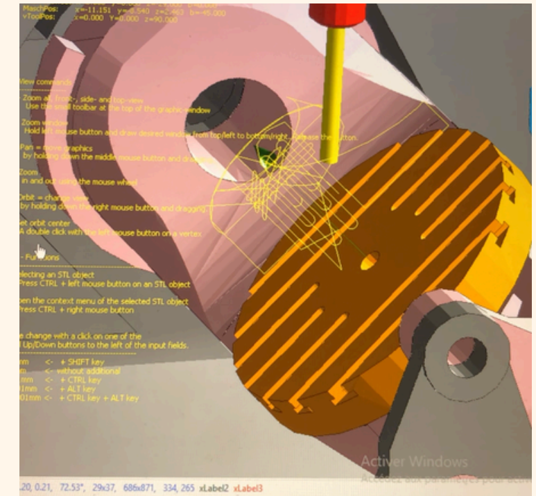
Carte Arduino méga et simulation d'usinage sur GRBL Gru
