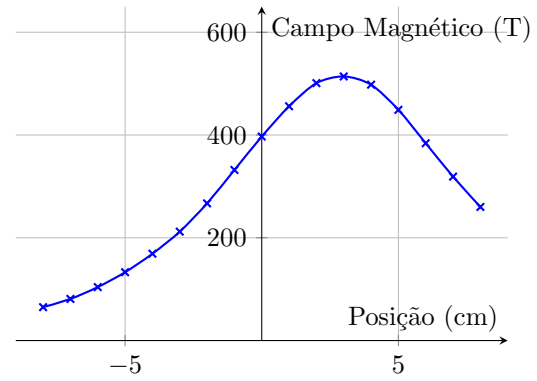
(b) Bobina da direita
