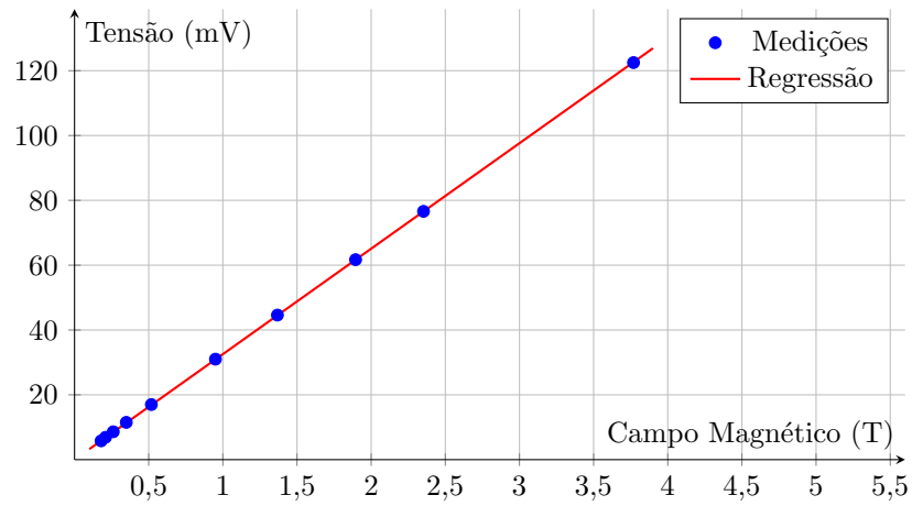
Figura 1: Calibração da sonda - Gráfico V-B
