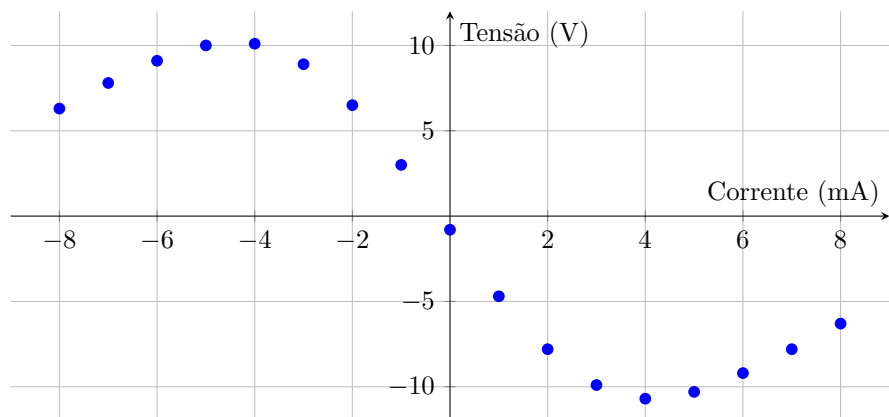
Figura 5: Gráfico V-I montagem 1 - caso a)
