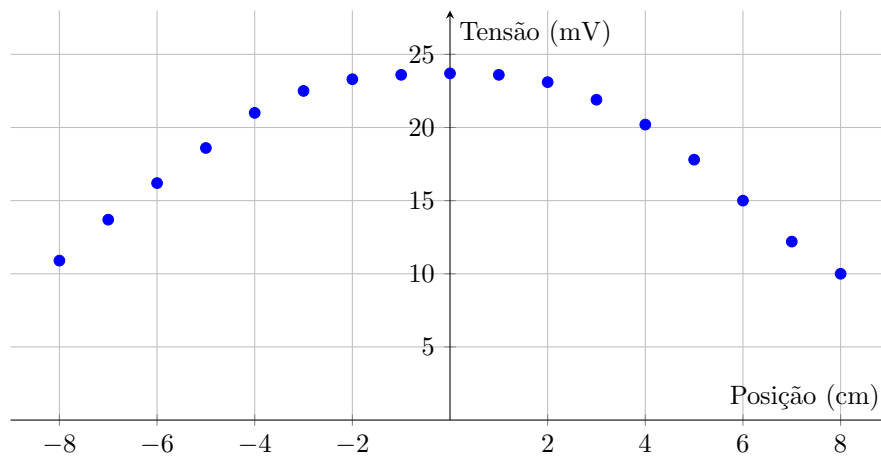
Figura 2: Gráfico - tensão ao longo das bobinas
