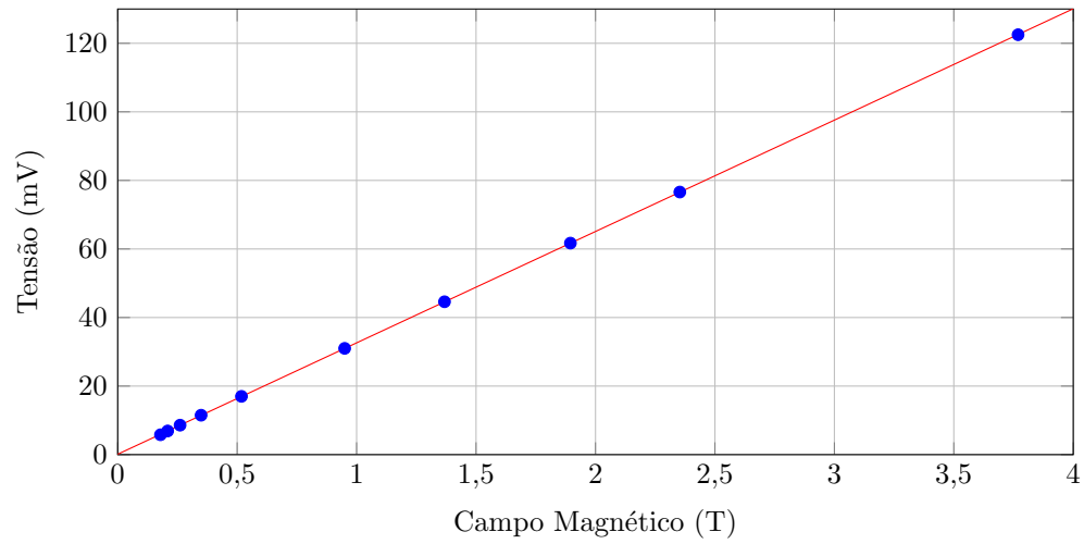
Figura 1: Calibração da sonda - Gráfico V-B
