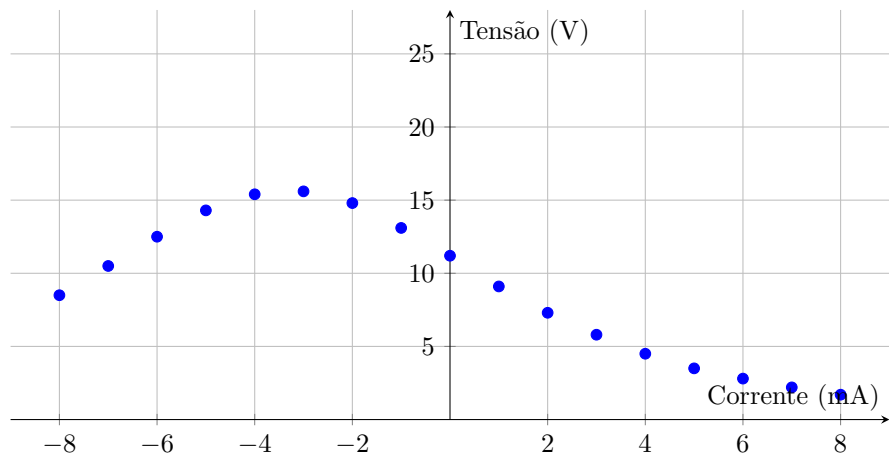
Figura 4: Gráfico V-I montagem 1 - caso a)
