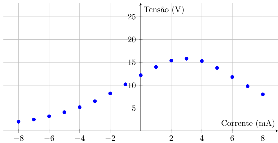
Figura 3: Gráfico V-I montagem 1 - caso a)
