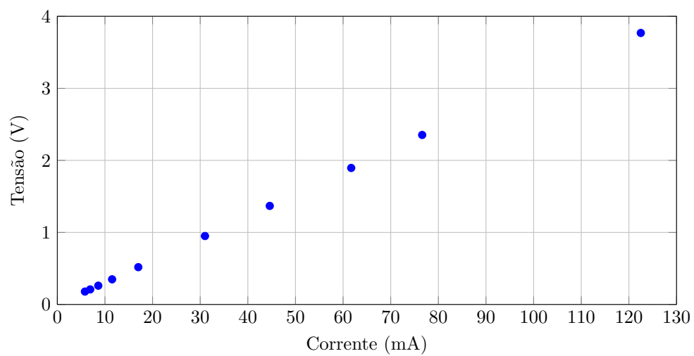
Figura 1: Gráfico V-I montagem 1 - caso a)
