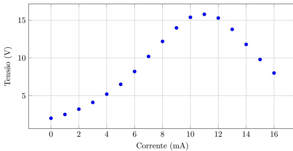
Figura 3: Gráfico V-I montagem 1 - caso a)
