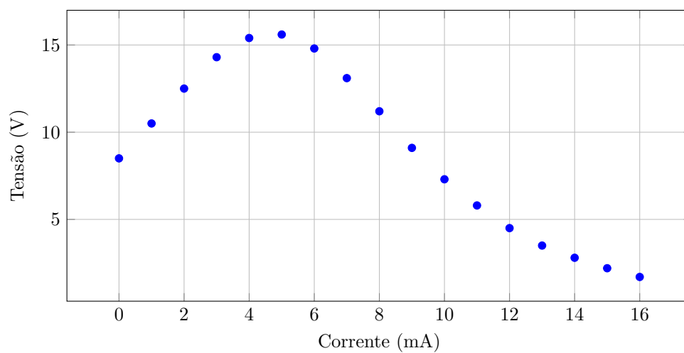
Figura 4: Gráfico V-I montagem 1 - caso a)
