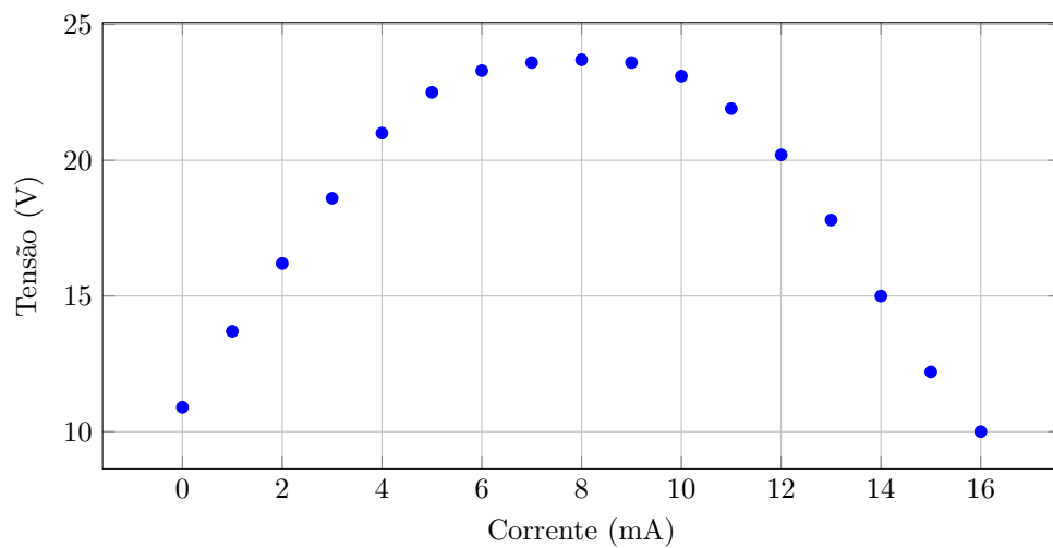
Figura 2: Gráfico V-I montagem 1 - caso a)
