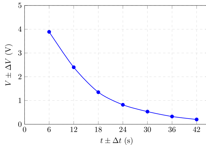
Figura 2: Tensão em função do tempo - Descarga
