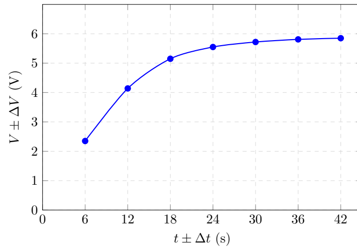
Figura 1: Tensão em função do tempo - Carga
