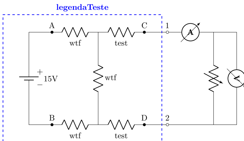
Figura 3: Montagem experimental
