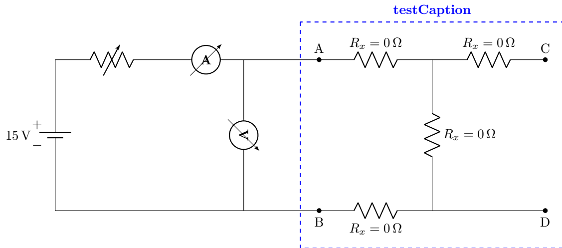
Figura 1: Montagem experimental
