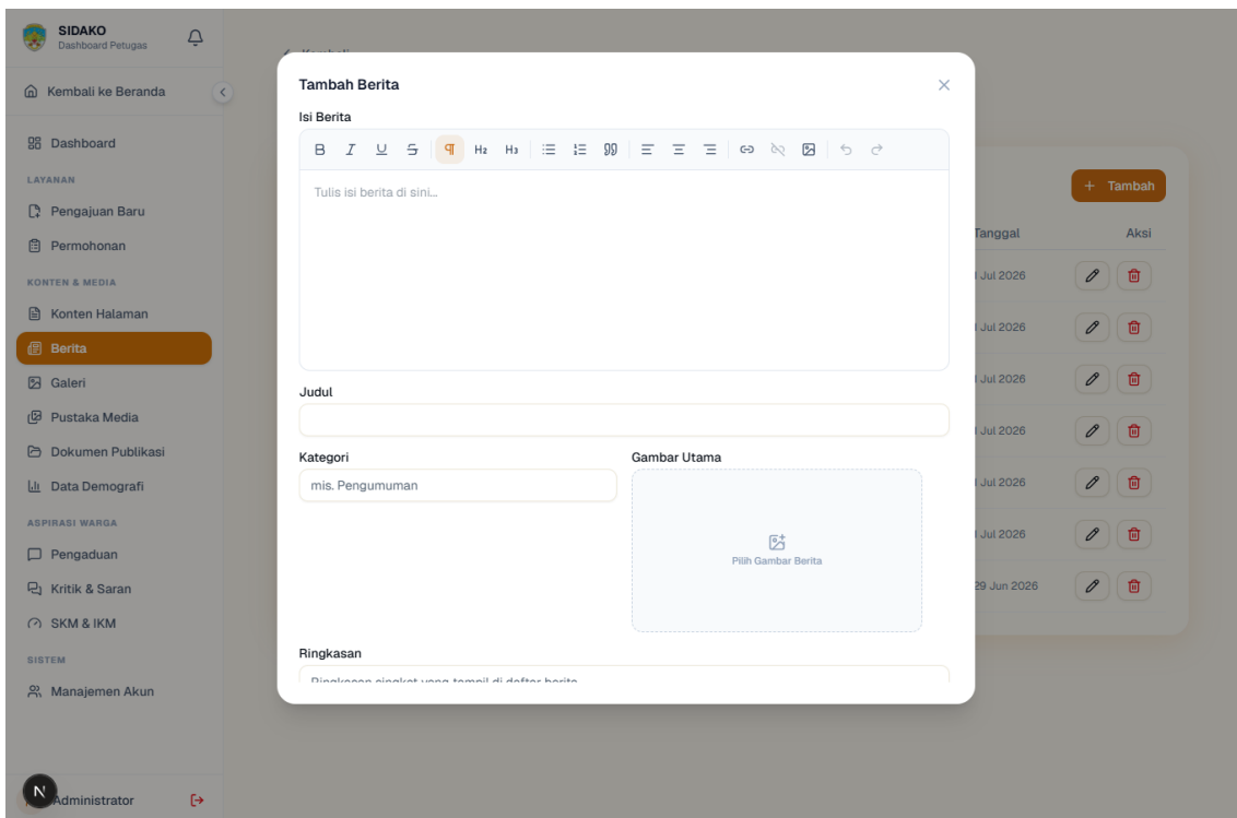
Editor berita — judul, kategori, konten Tiptap, gambar utama, dan saklar publish.
