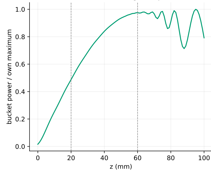
(d) fixed-bucket integrated power
