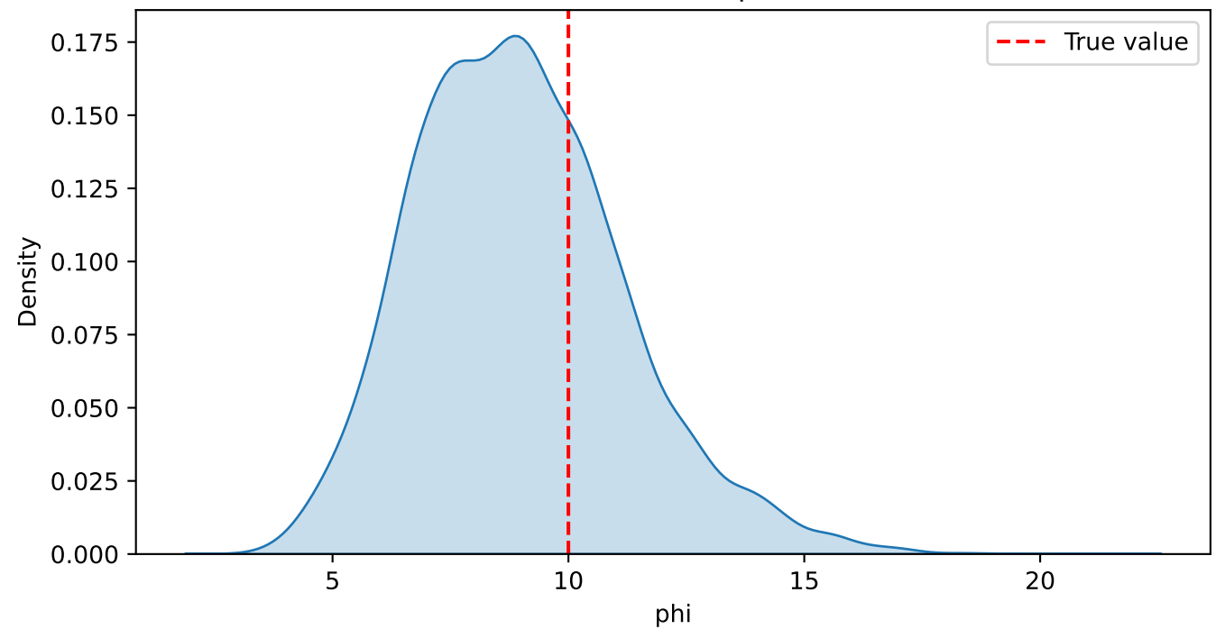
Posterior of phi
