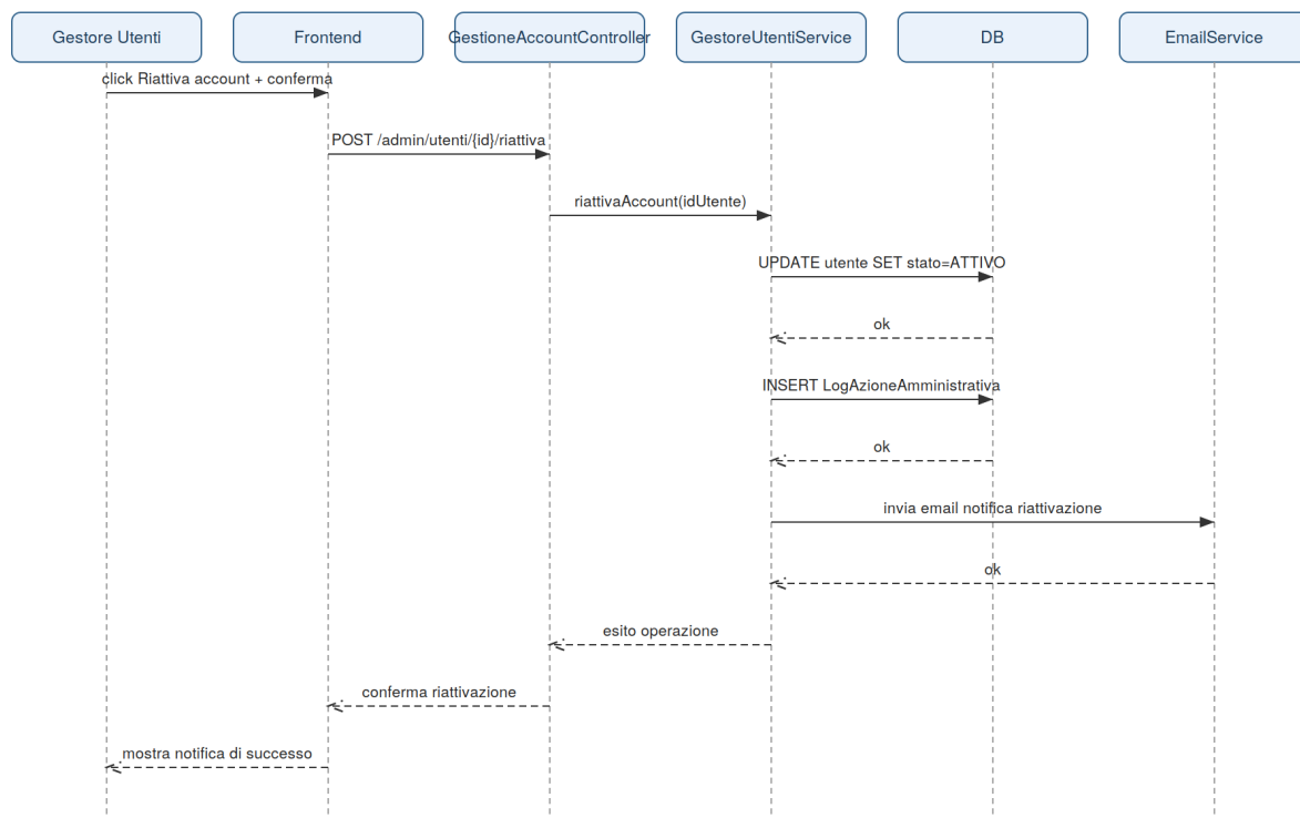
Sequence Diagram – UC_24 Riattivazione Account
