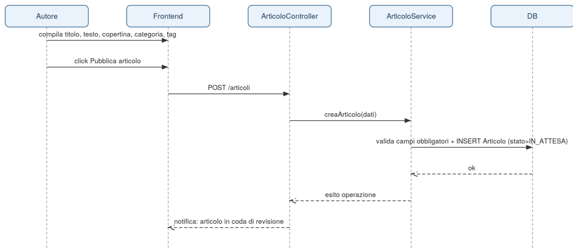
Sequence Diagram – UC_15 Creazione e Pubblicazione Articolo
