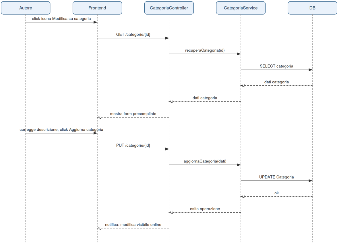
Sequence Diagram – UC_14 Modifica Categoria
