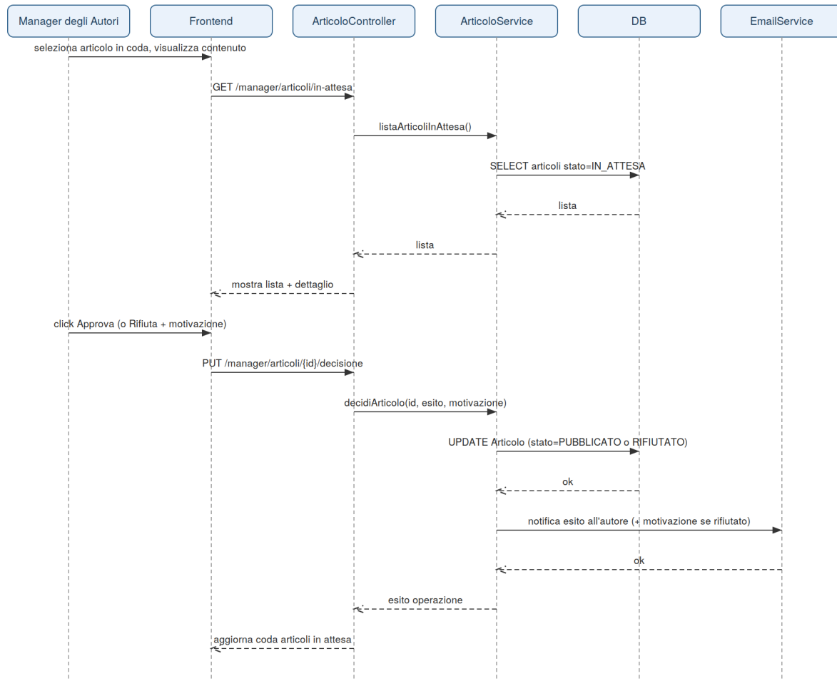
Sequence Diagram – UC_21 Approvazione / Rifiuto Articolo
