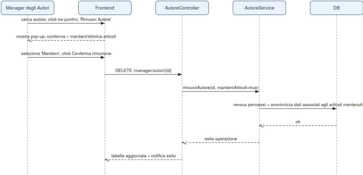
Sequence Diagram – UC_11 Rimozione Autore
