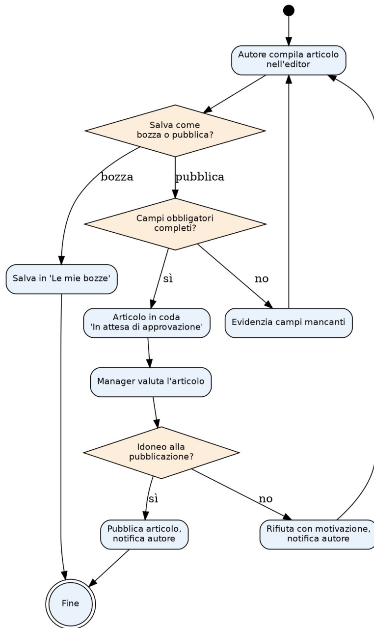
Activity Diagram - Pubblicazione Articolo
