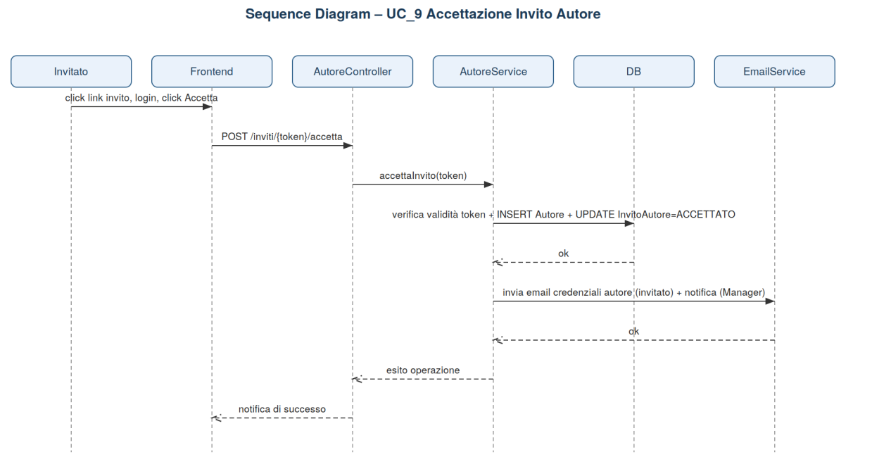
Sequence Diagram – UC_9 Accettazione Invito Autore
