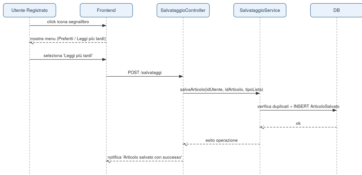
Sequence Diagram – UC_6 Salvataggio Articolo (Preferiti/Leggi più tardi)
