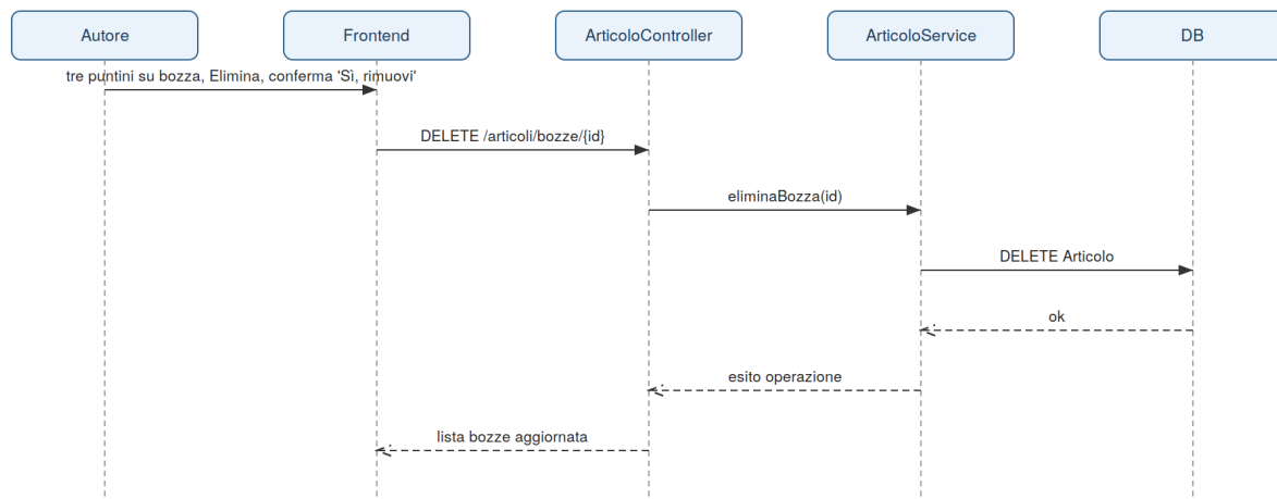
Sequence Diagram – UC_18 Cancellazione Bozza
