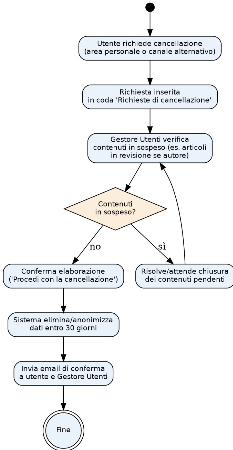
Activity Diagram - Cancellazione Account
