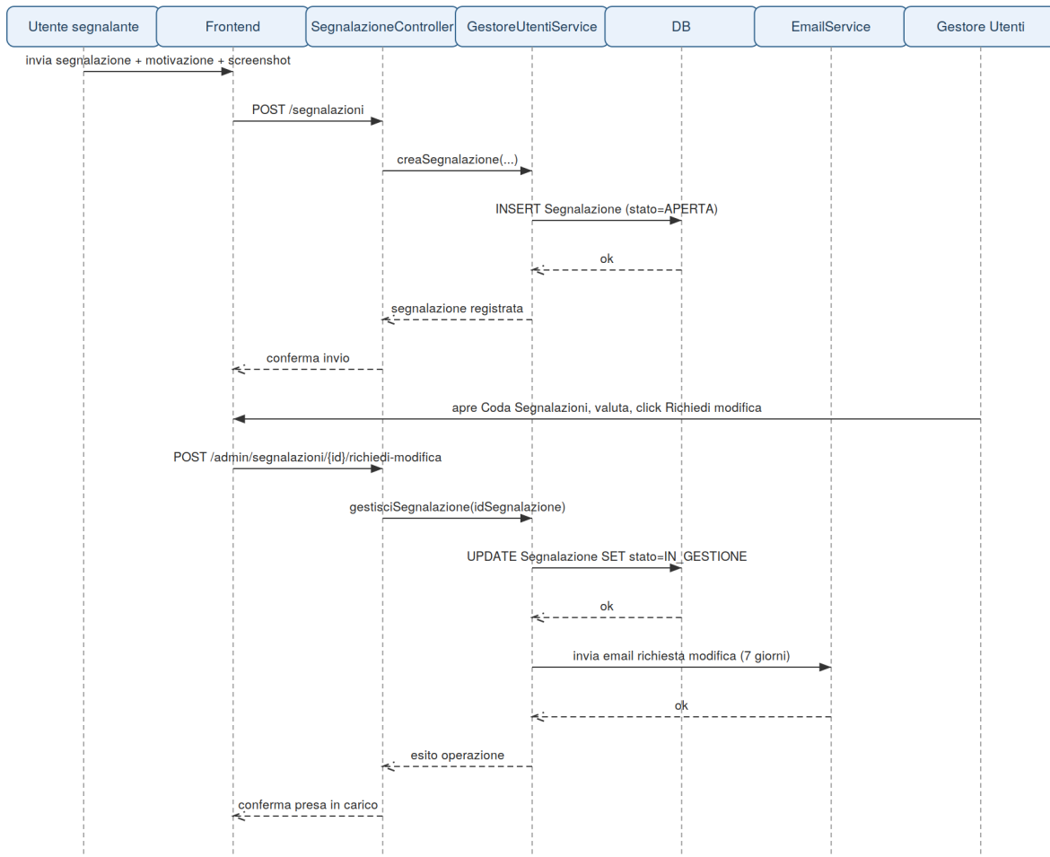
Sequence Diagram – UC_26 Gestione di una Segnalazione
