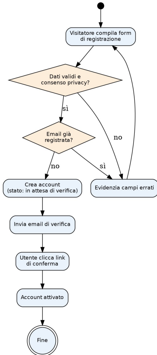
Activity Diagram - Registrazione
