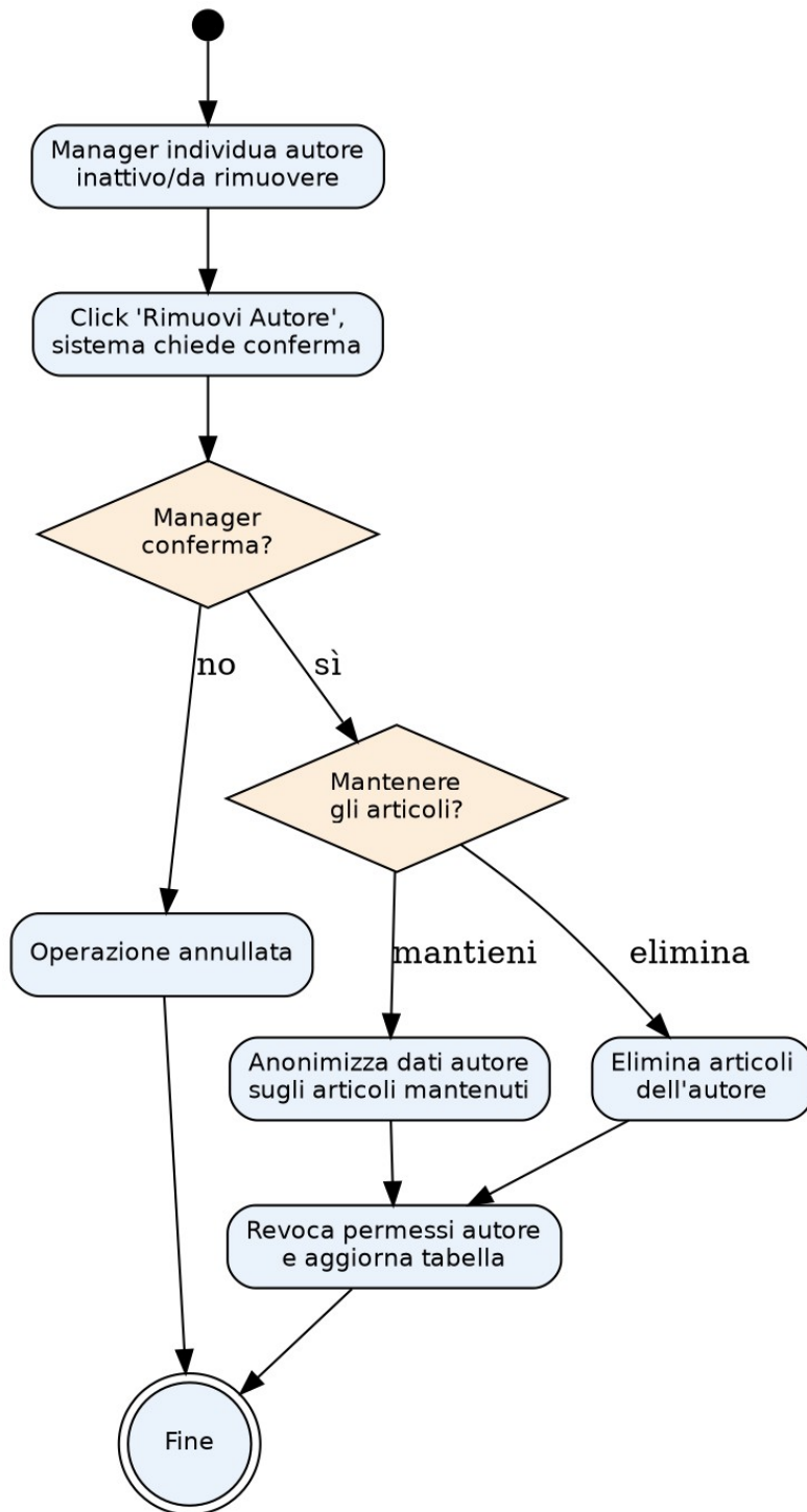
Activity Diagram - Rimozione Autore
