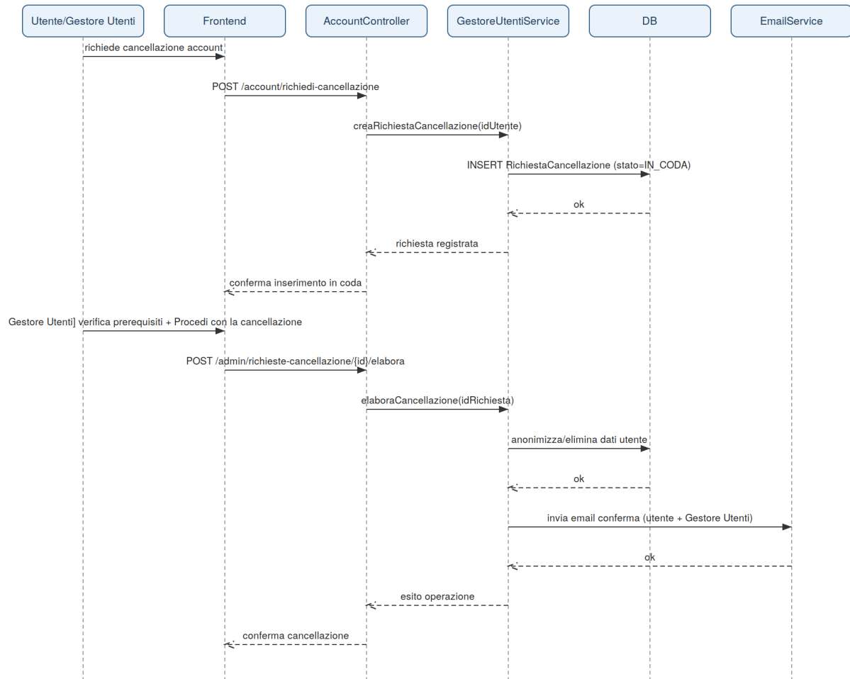
Sequence Diagram – UC_25 Cancellazione Account (Diritto all'oblio)
