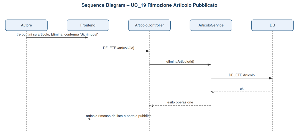
Sequence Diagram – UC_19 Rimozione Articolo Pubblicato
