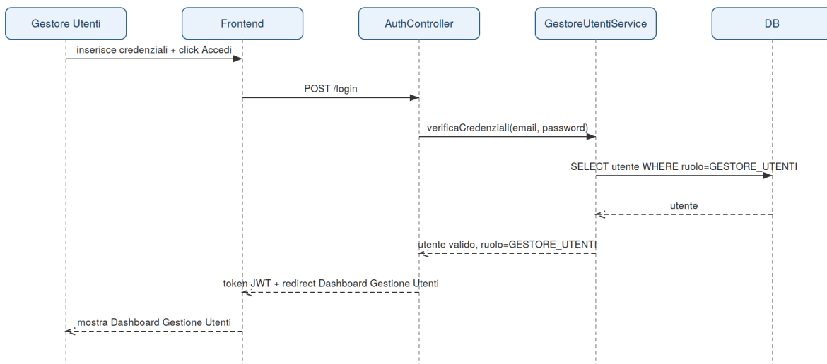
Sequence Diagram – UC_22 Autenticazione Gestore Utenti
