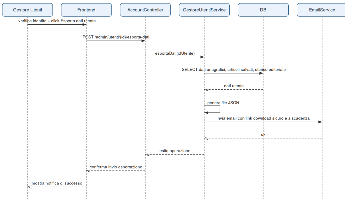
Sequence Diagram – UC_27 Esportazione Assistita dei Dati Personali
