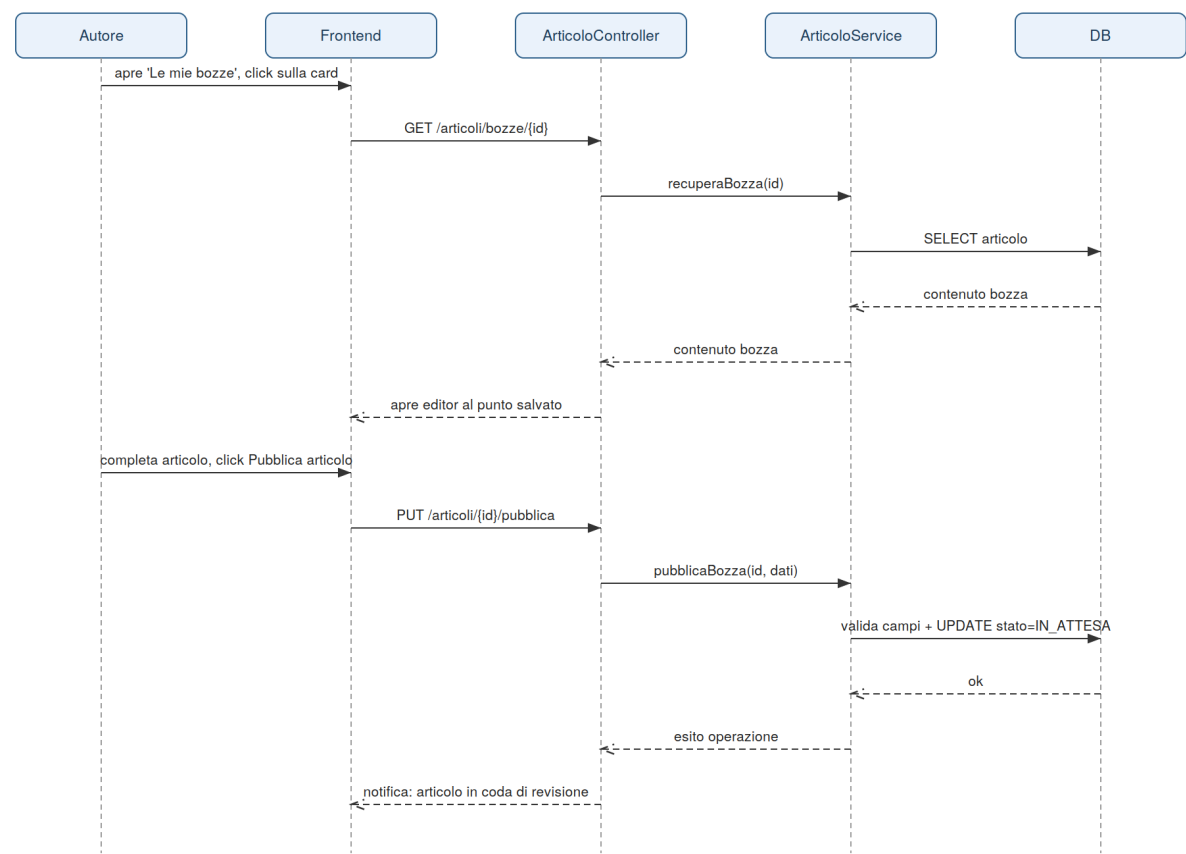
Sequence Diagram – UC_17 Ripresa Bozza e Pubblicazione
