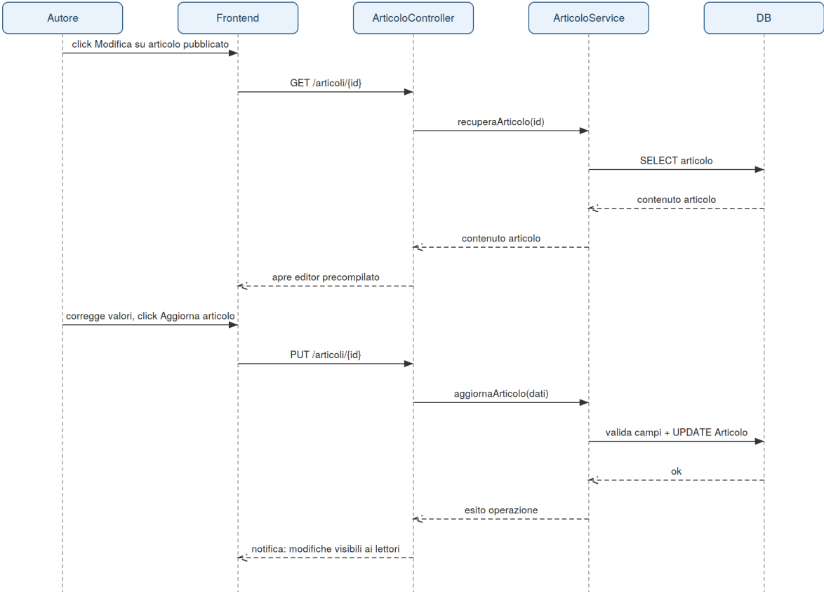
Sequence Diagram – UC_20 Modifica Articolo Pubblicato
