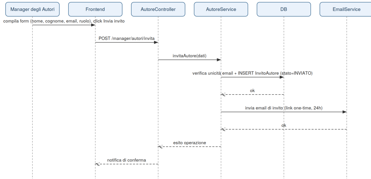
Sequence Diagram – UC_8 Aggiunta Autore
