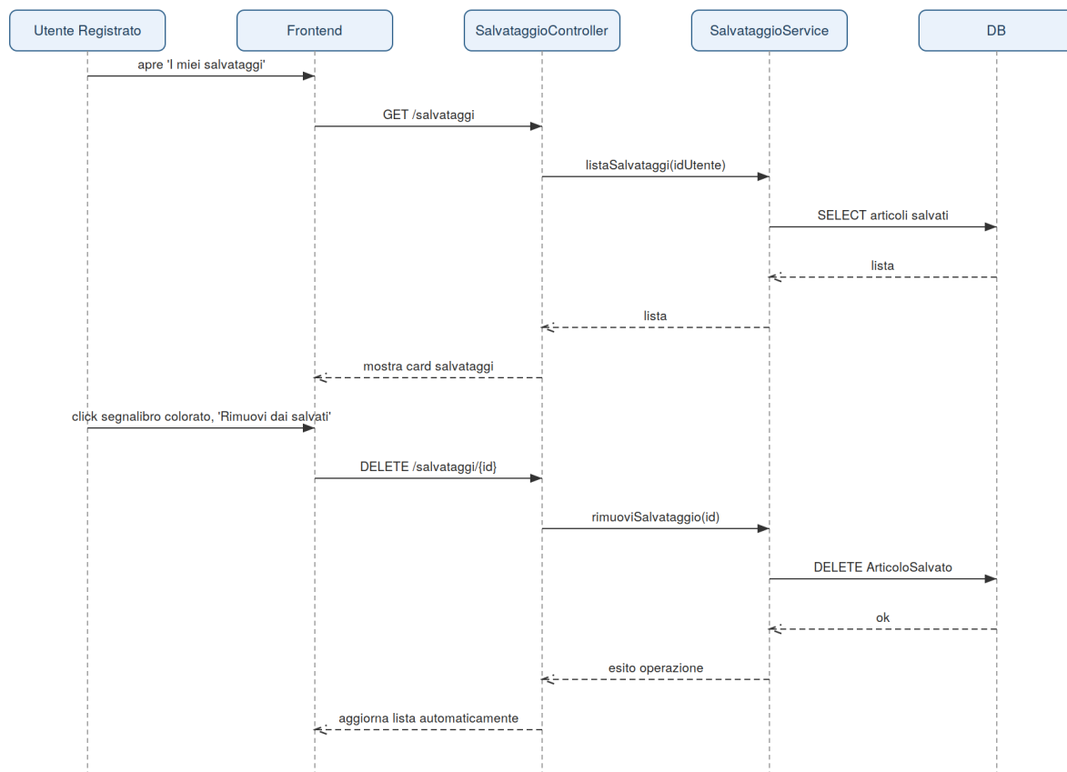
Sequence Diagram – UC_7 Rimozione Articolo dai Salvati
