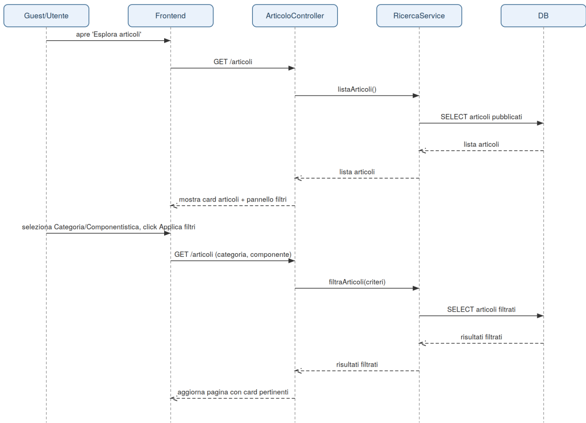
Sequence Diagram – UC_5 Ricerca e Filtro Articoli
