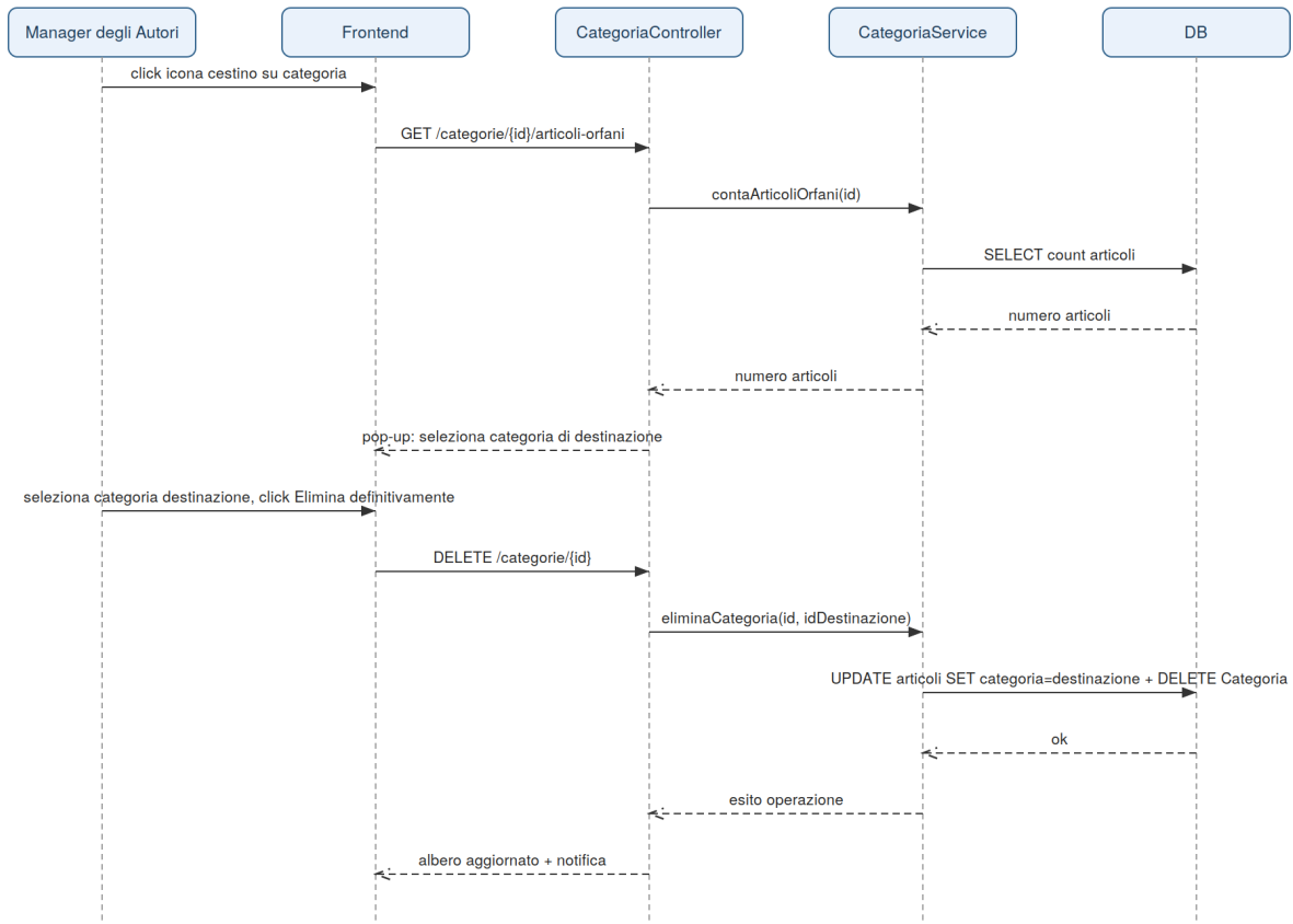
Sequence Diagram – UC_13 Rimozione Categoria
