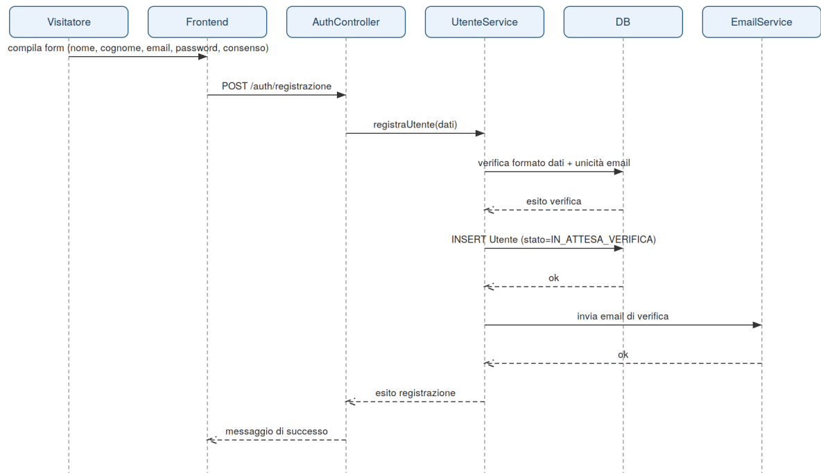
Sequence Diagram – UC_1 Registrazione Utente
