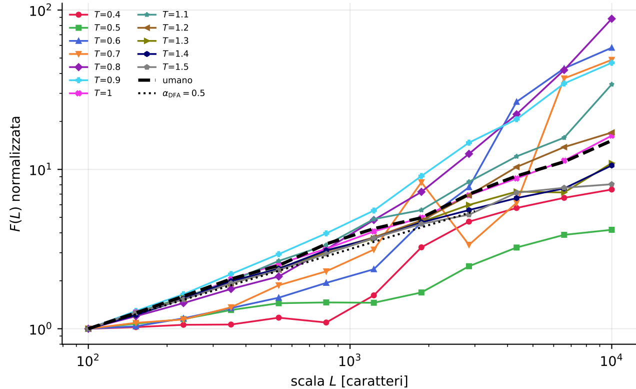
DFA sui caratteri — Qwen2.5-1.5B (cfr. [L] Fig. 4A)
