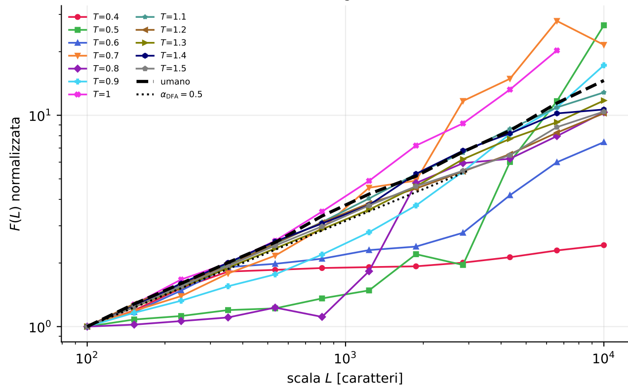
DFA sui caratteri, detrending di ordine 2 — Qwen2.5-3B
