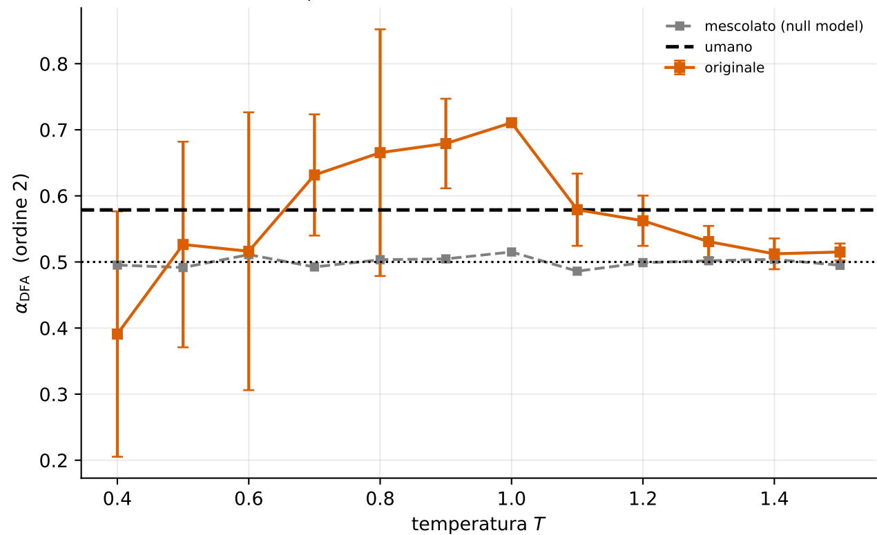
Esponente DFA di ordine 2 — Qwen2.5-3B
