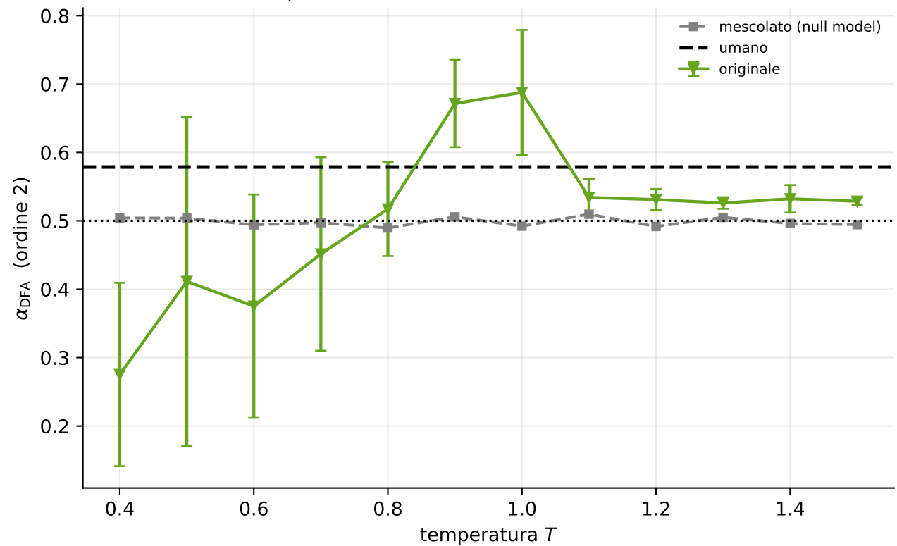
Esponente DFA di ordine 2 — Qwen3.5-4B-Base
