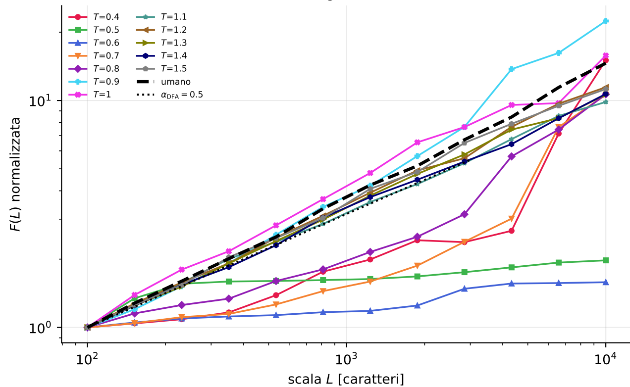
DFA sui caratteri, detrending di ordine 2 — Qwen3.5-4B-Base
