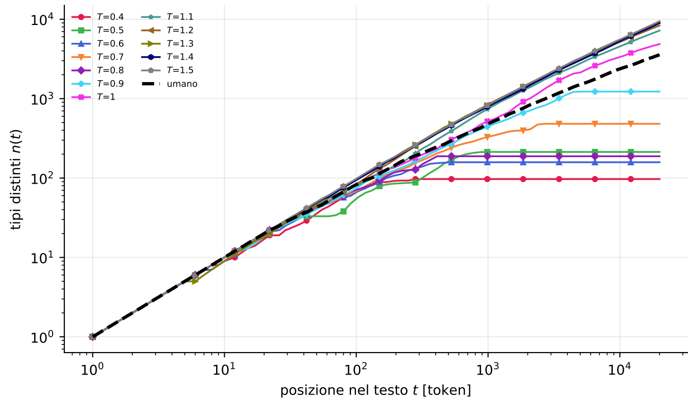
Curve di Heaps — Qwen2.5-3B (cfr. [Z] Fig. 3, [L] Fig. 3A)
