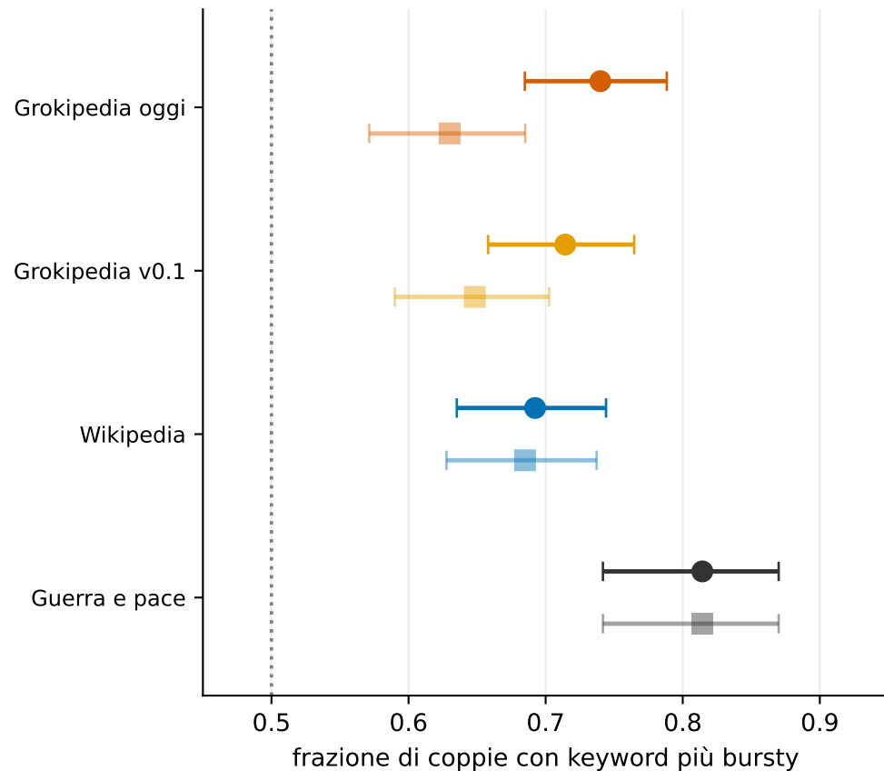
B. Il test interno della Fig. 5.3A quadrati: lista originaria; cerchi: lista estesa
