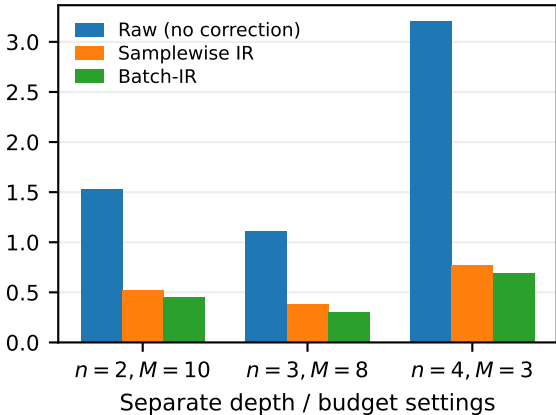
Value MAE
