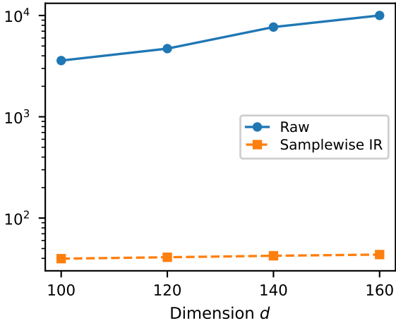
Generator MSE
