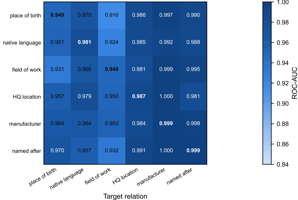
Llama-3.1-70B (layer 39, depth 50%)
