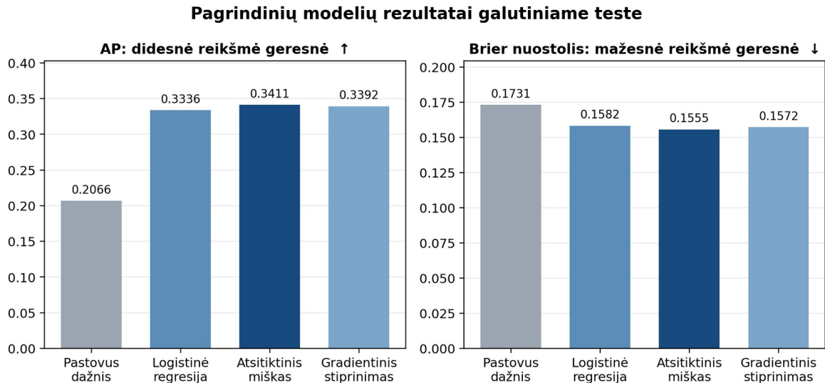
2 pav. Pagrindinių modelių AP ir Brier palyginimas
