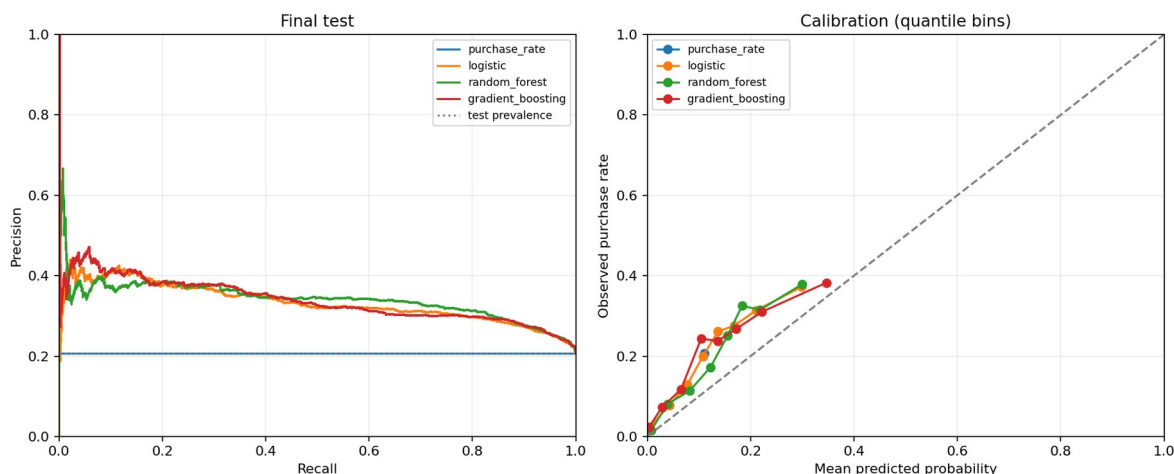
3 pav. Precision–recall ir tikimybių kalibracijos kreivės
