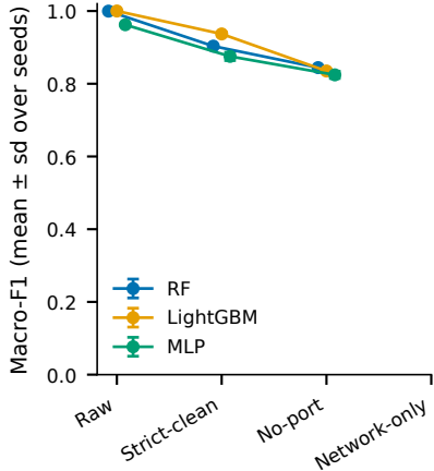
Edge-IIoTset
