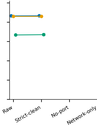
CICIoT2023
