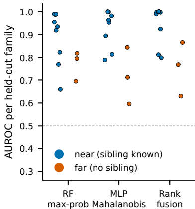
Edge-IIoTset
