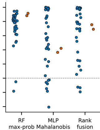
CICIoT2023
