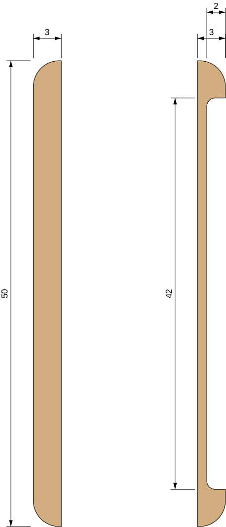
Vue de face pleine - 1:4
