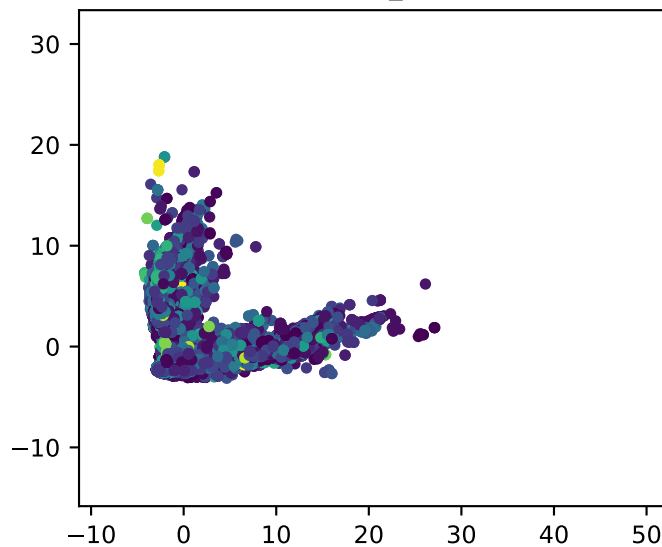
conv_4
