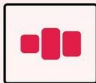
center
