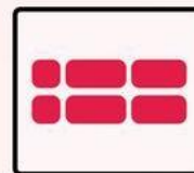
center
