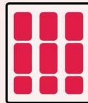
column-reverse
