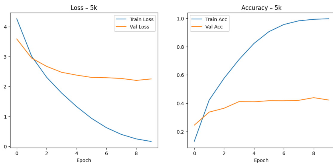
3.87. ábra. 5k adathalmazon történő tanítás grafikonja DenseNet121 modellen.
