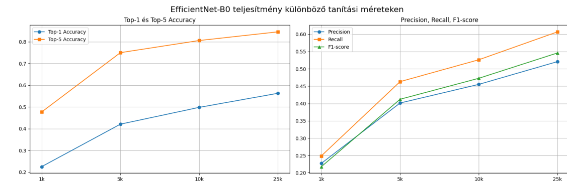
3.102. ábra. Összehasonlító metrika grafikon a EfficientNet-B0 iteratív tanításáról.
