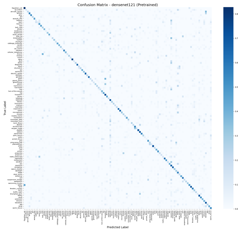
3.4. ábra. DenseNet121 tanítás nélküli normalizált Confusion Mátrix
