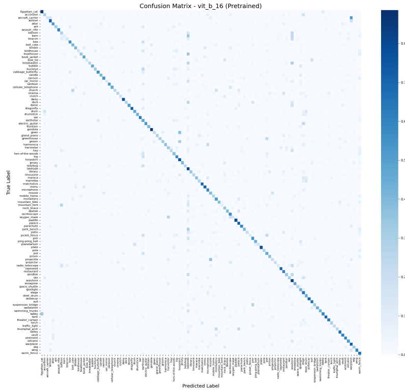
3.10. ábra. ViT-B-16 tanítás nélküli normalizált Confusion Mátrix
