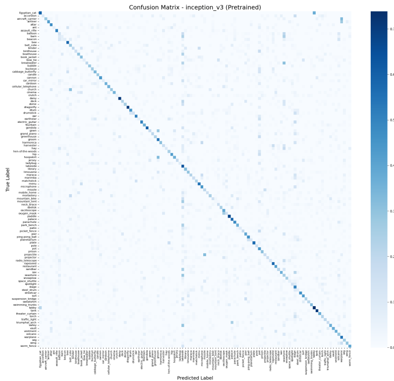
3.12. ábra. Inception-v3 tanítás nélküli normalizált Confusion Mátrix
