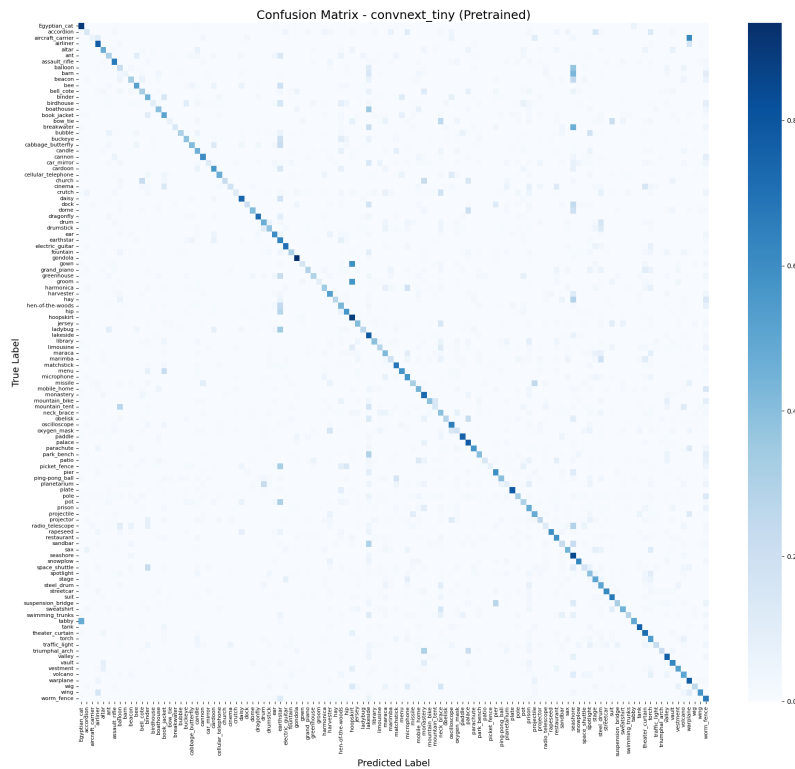
3.8. ábra. ConvNeXt-Tiny tanítás nélküli normalizált Confusion Mátrix
