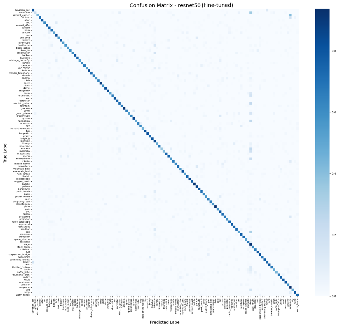
3.21. ábra. ResNet50 teljes tanítás utáni normalizált Confusion Mátrix
