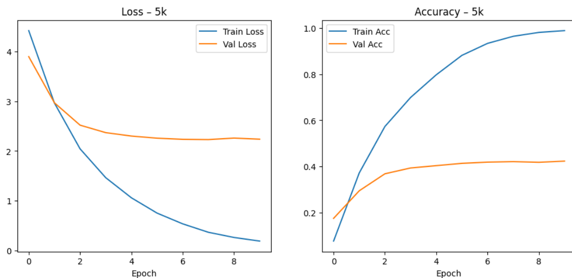
3.94. ábra. 5k adathalmazon történő tanítás grafikonja EfficientNet-B0 modellen.
