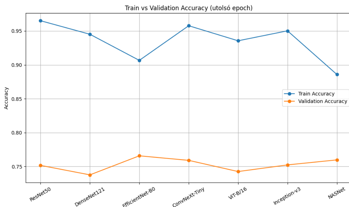
3.76. ábra. A Train és Validation accuracy alakulása modellenként.
