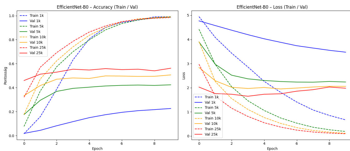
3.98. ábra. Összehasonlító grafikon a EfficientNet-B0 iteratív tanításáról 10 EPOCH-on keresztül.
