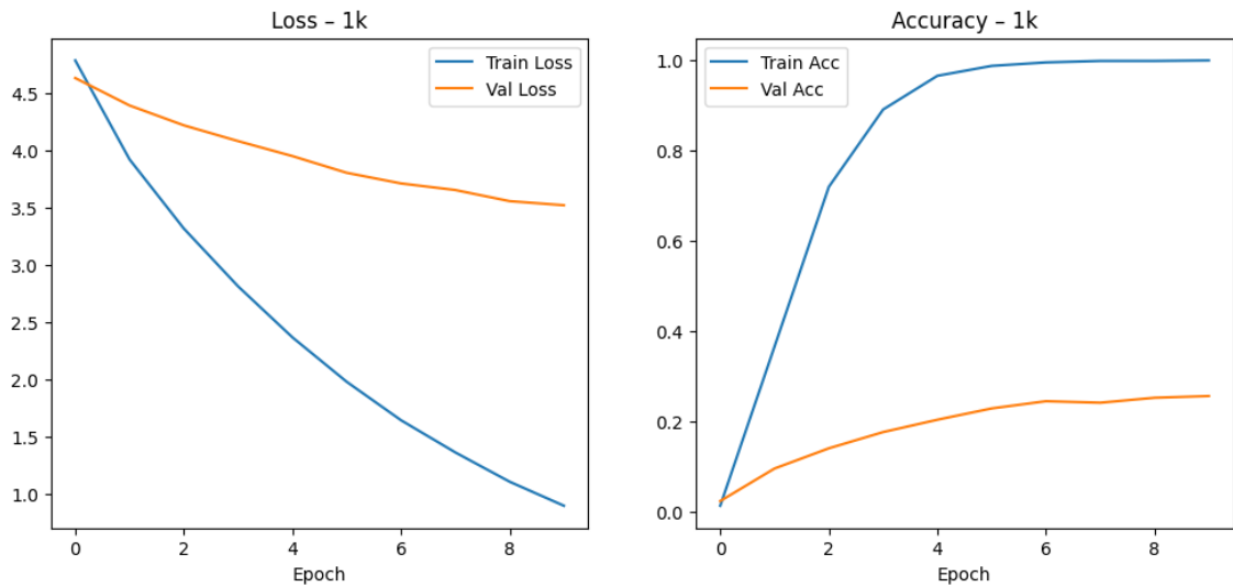
3.86. ábra. 1k adathalmazon történő tanítás grafikonja DenseNet121 modellen.
