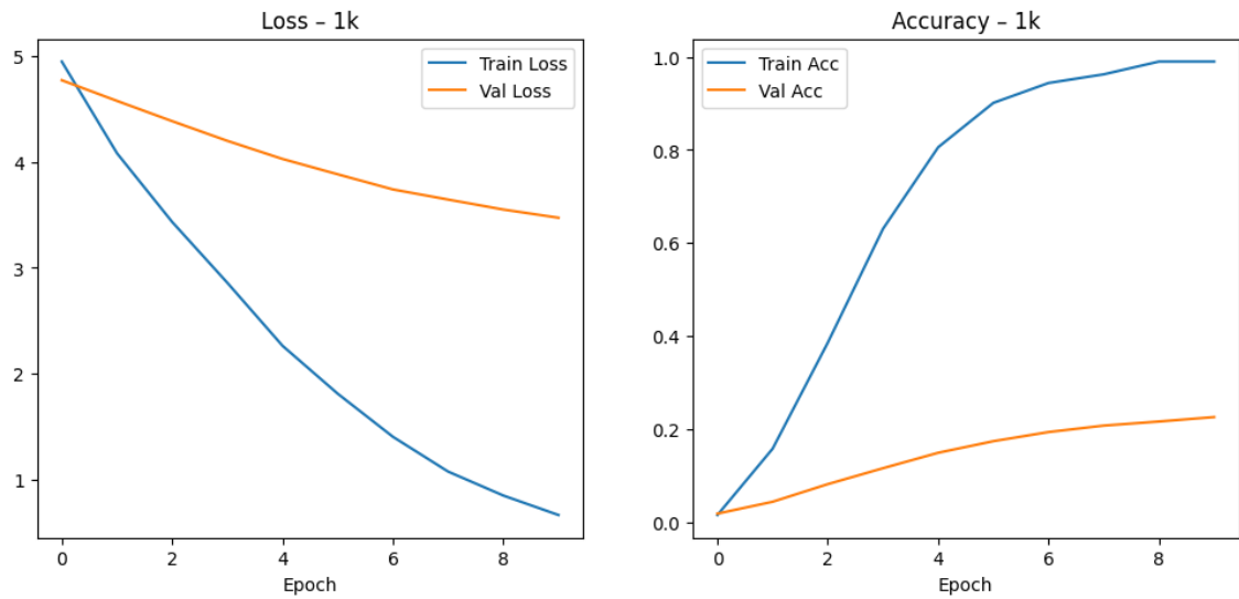
3.93. ábra. 1k adathalmazon történő tanítás grafikonja EfficientNet-B0 modellen.
