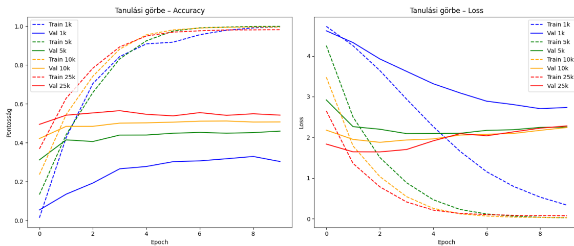
3.84. ábra. Összehasonlító grafikon a ResNet50 iteratív tanításáról 10 EPOCH-on keresztül.
