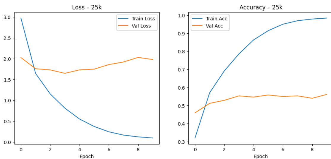
3.96. ábra. 25k adathalmazon történő tanítás grafikonja EfficientNet-B0 modellen.
