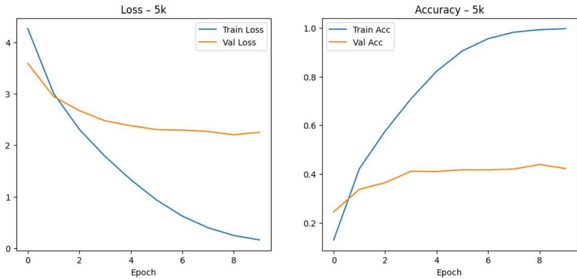
3.87. ábra. 5k adathalmazon történő tanítás grafikonja DenseNet121 modellen.
