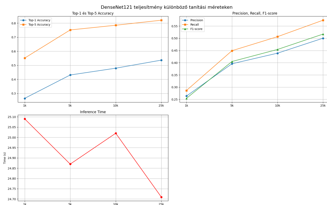
3.90. ábra. Összehasonlító grafikon a DenseNet121 iteratív tanításáról.
