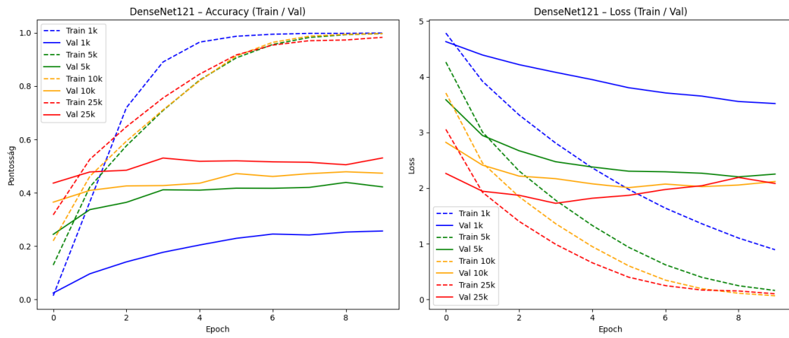
3.91. ábra. Összehasonlító grafikon a DenseNet121 iteratív tanításáról 10 EPOCH-on keresztül.
