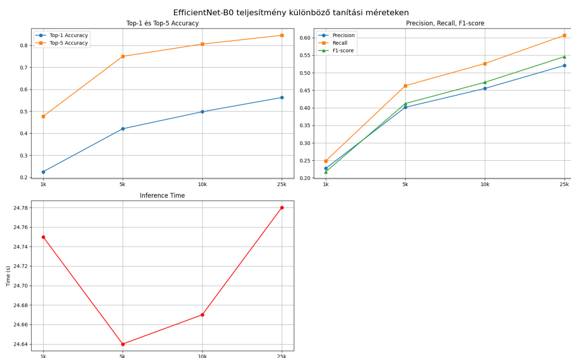
3.97. ábra. Összehasonlító grafikon a EfficientNet-B0 iteratív tanításáról.
