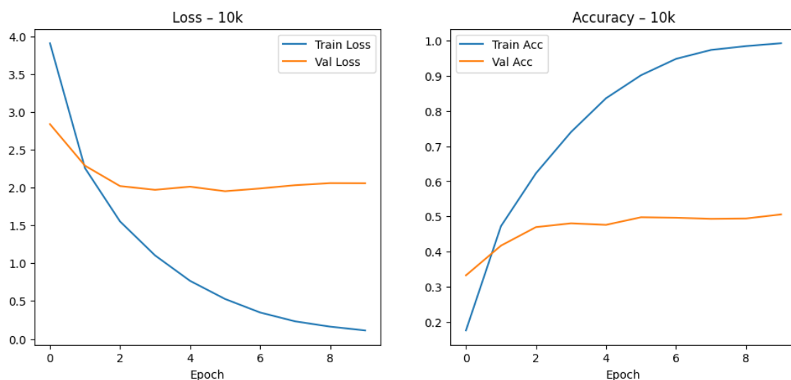
3.95. ábra. 10k adathalmazon történő tanítás grafikonja EfficientNet-B0 modellen.
