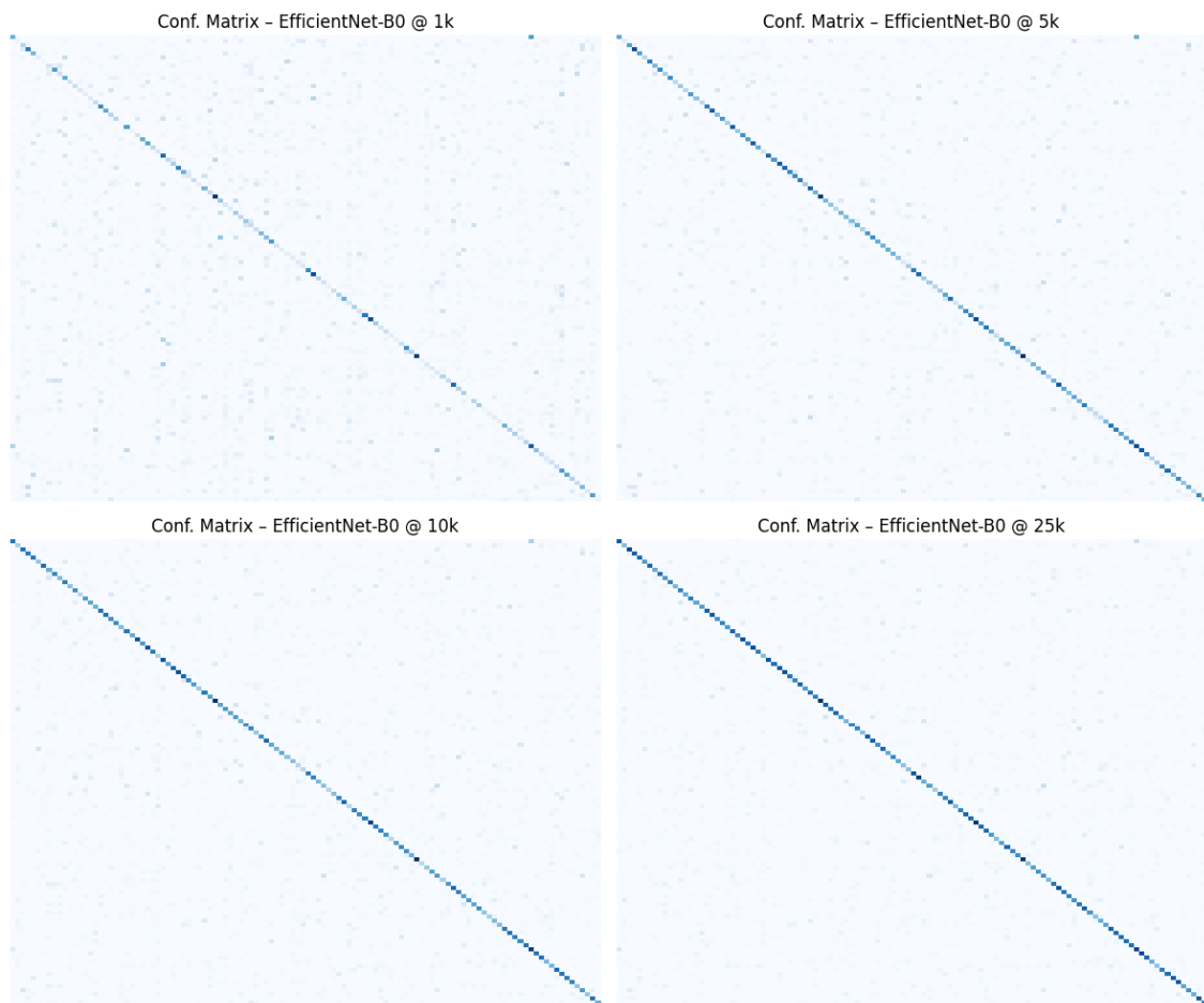
3.99. ábra. Összehasonlító Confusion Matrix a EfficientNet-B0 iteratív tanításáról 10 EPOCH-on keresztül.
