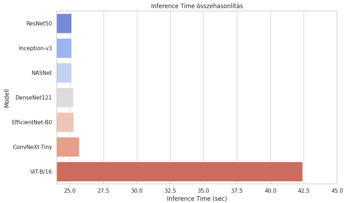
3.69. ábra. Futási idők összehasonlítása teljes tanítás után a teszt halmazon.
