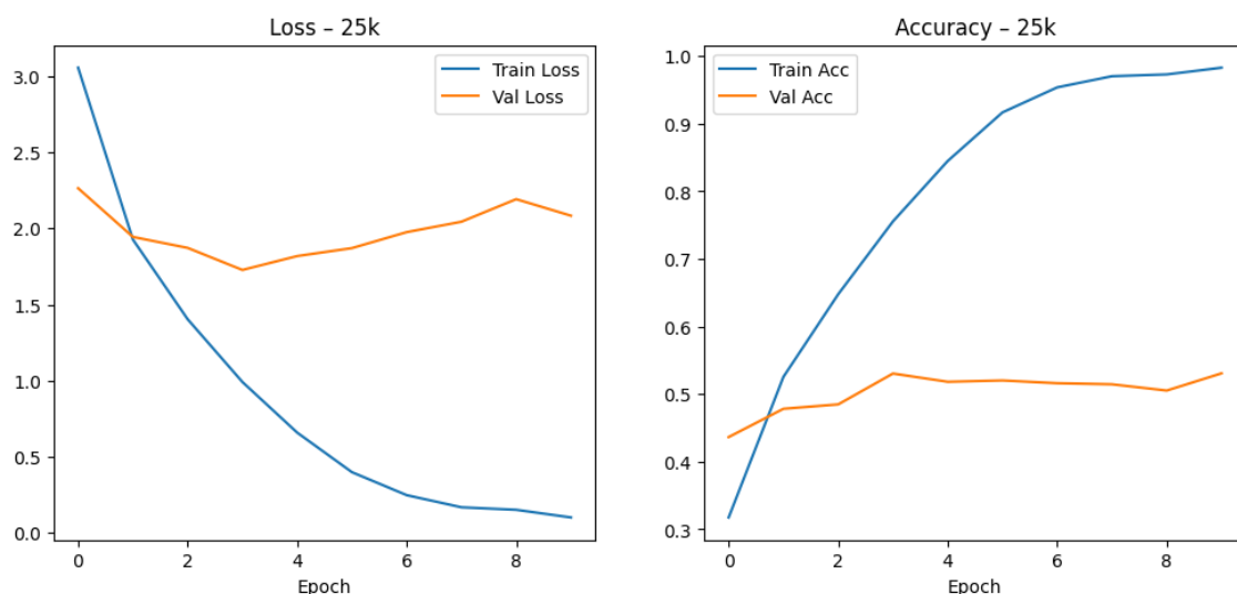
3.89. ábra. 25k adathalmazon történő tanítás grafikonja DenseNet121 modellen.
