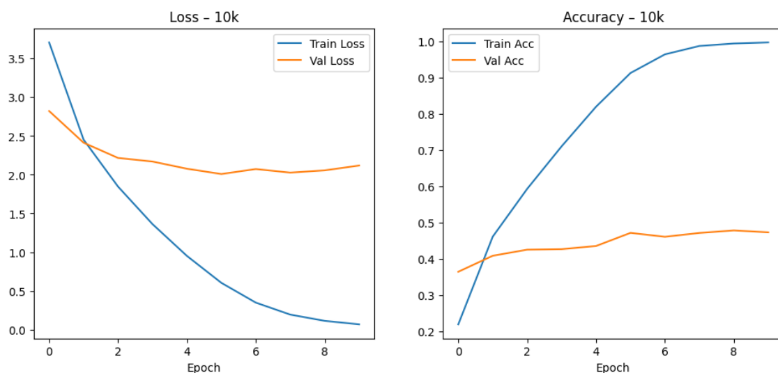
3.88. ábra. 10k adathalmazon történő tanítás grafikonja DenseNet121 modellen.
