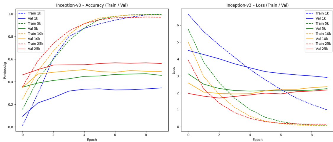
3.131. ábra. Összehasonlító grafikon a Inception-v3 iteratív tanításáról 10 EPOCH-on keresztül.
