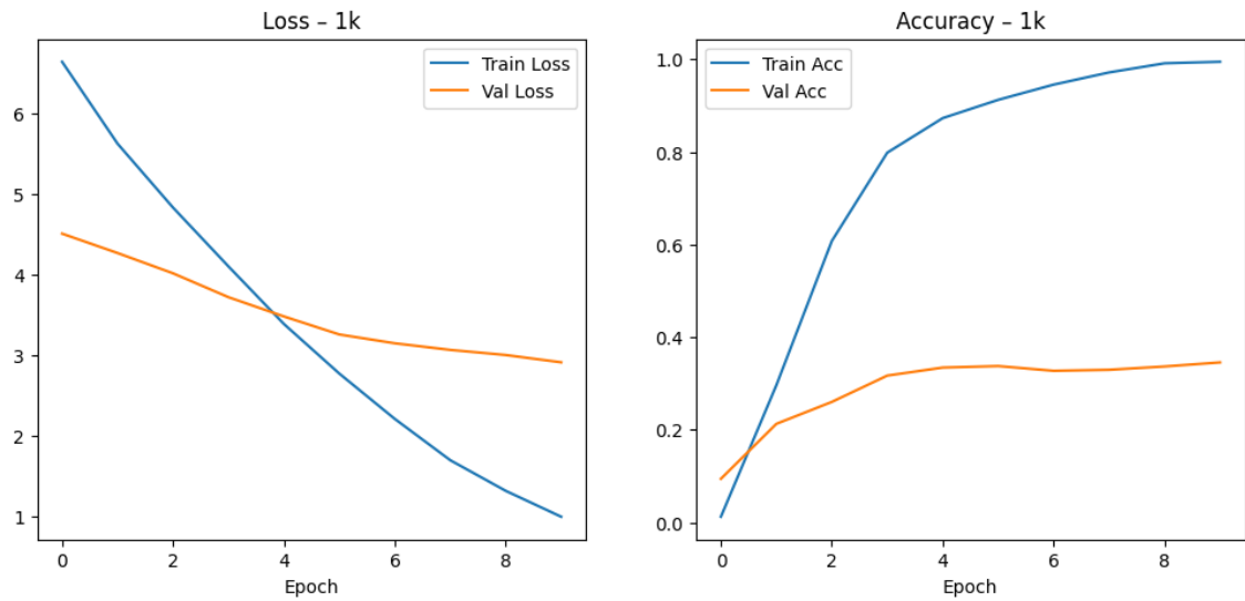
3.124. ábra. 1k adathalmazon történő tanítás grafikonja Inception-v3 modellen.
