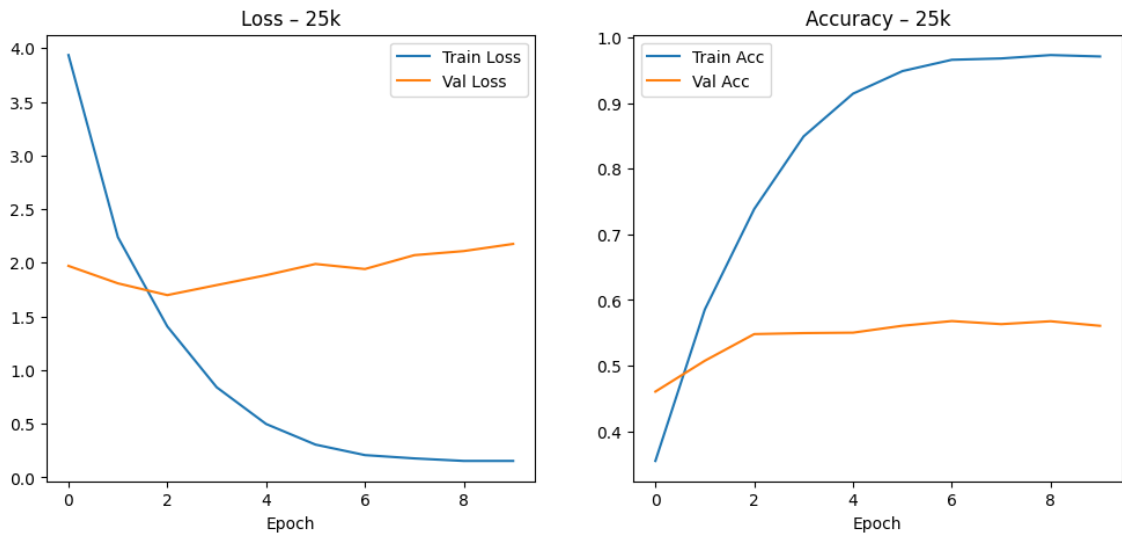
3.127. ábra. 25k adathalmazon történő tanítás grafikonja Inception-v3 modellen.
