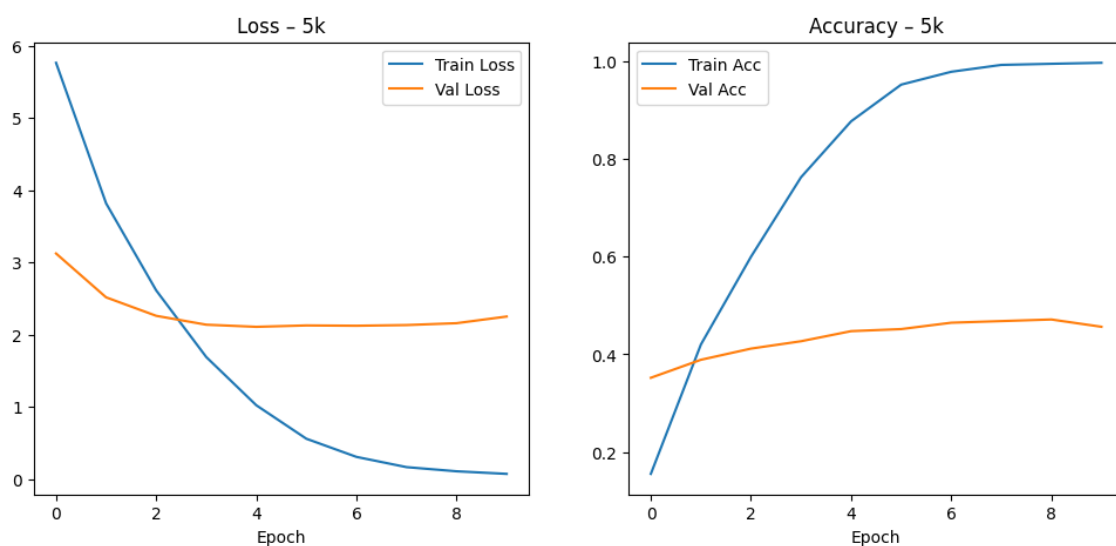
3.125. ábra. 5k adathalmazon történő tanítás grafikonja Inception-v3 modellen.
