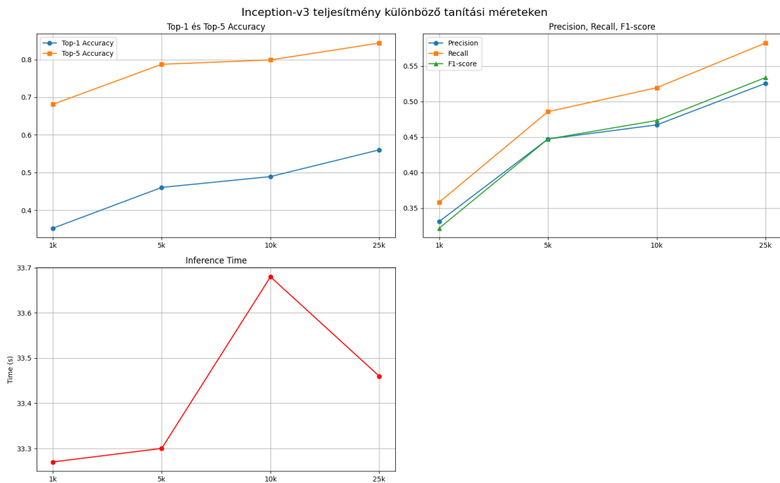
3.128. ábra. Összehasonlító grafikon a Inception-v3 iteratív tanításáról.
