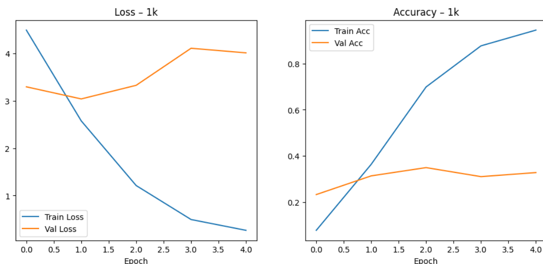
3.133. ábra. 1k adathalmazon történő tanítás grafikonja NASNet modellen.
