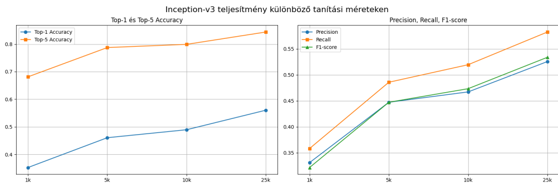
3.129. ábra. Összehasonlító metrika grafikon a Inception-v3 iteratív tanításáról.
