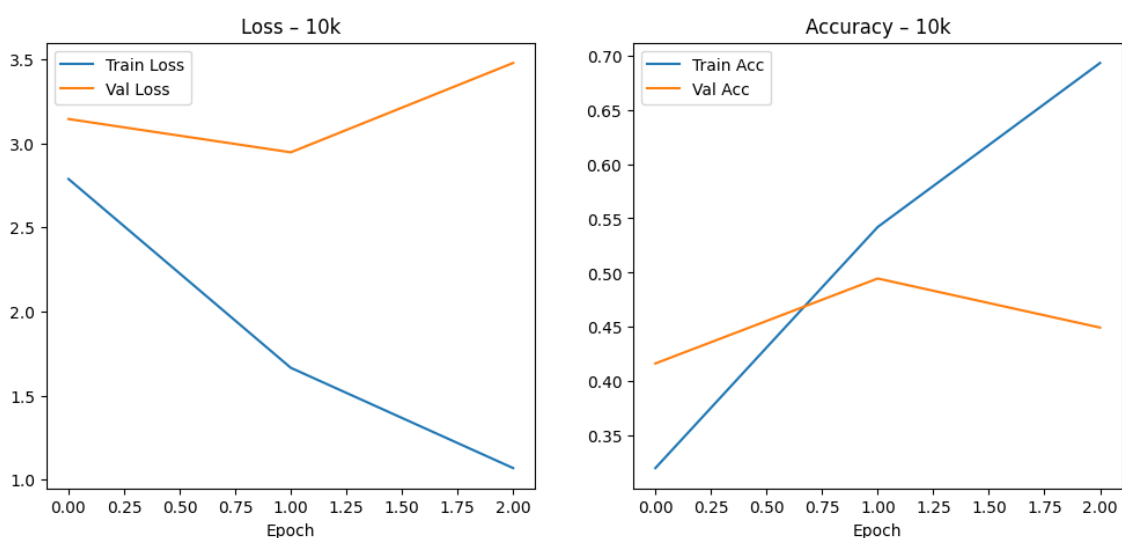
3.135. ábra. 10k adathalmazon történő tanítás grafikonja NASNet modellen.
