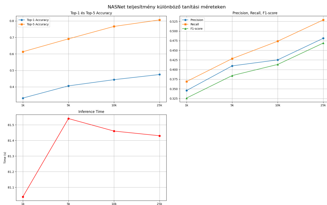
3.137. ábra. Összehasonlító grafikon a NASNet iteratív tanításáról.
