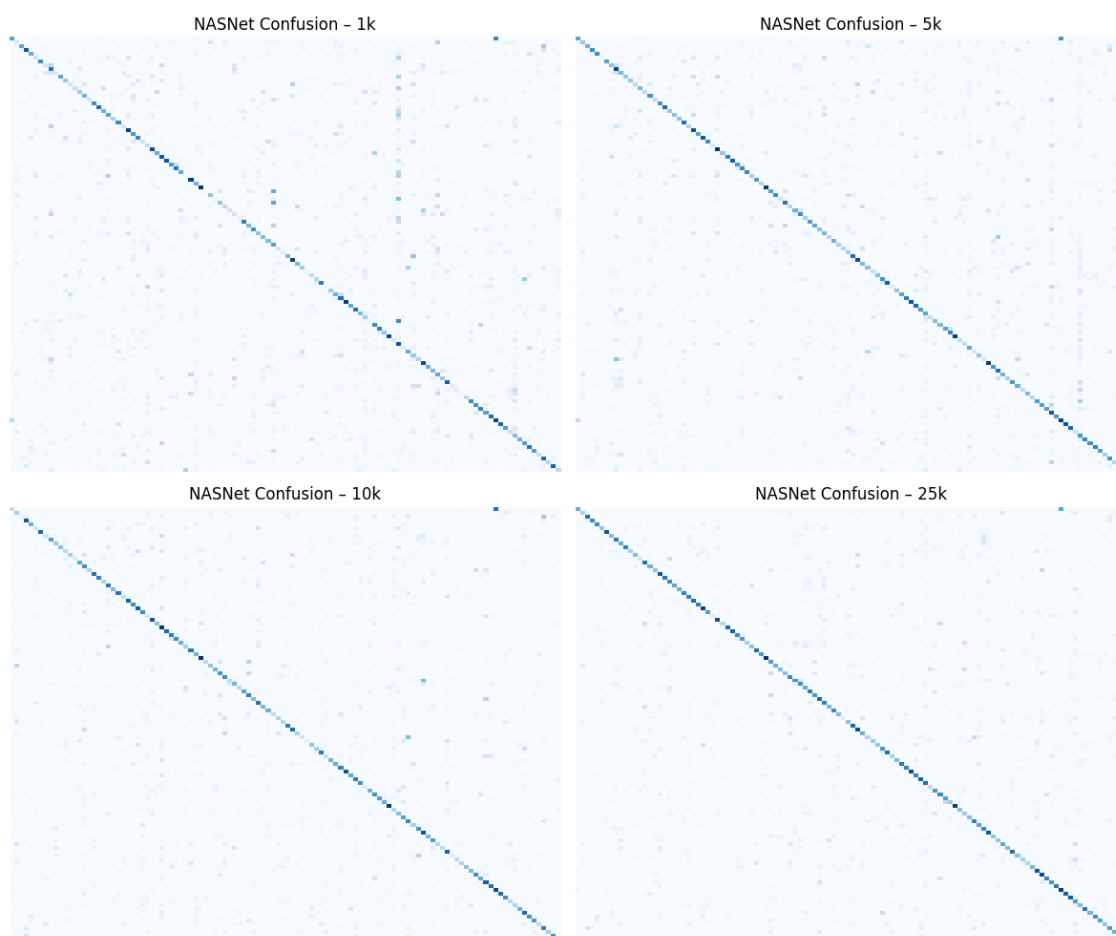
3.141. ábra. Összehasonlító Confusion Matrix a NASNet iteratív tanításáról 10 EPOCH-on keresztül.
