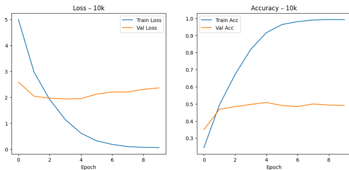
3.126. ábra. 10k adathalmazon történő tanítás grafikonja Inception-v3 modellen.
