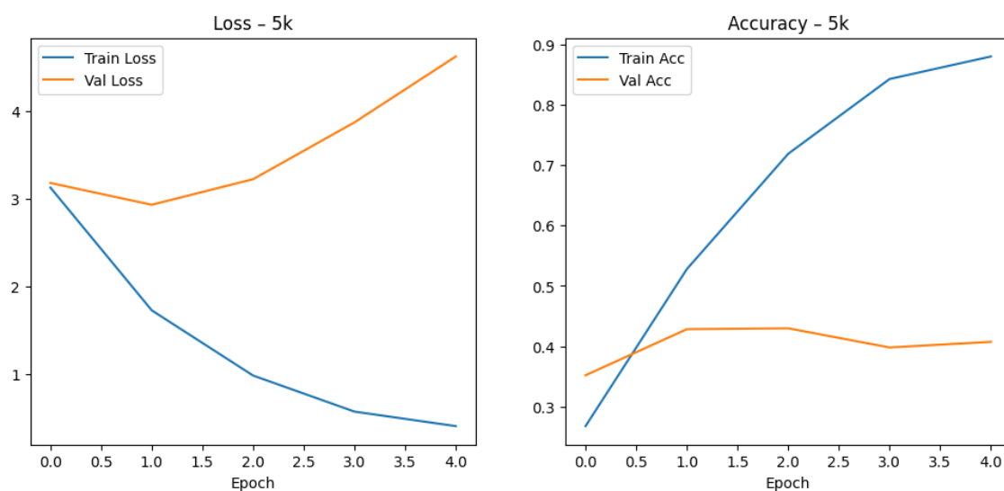
3.134. ábra. 5k adathalmazon történő tanítás grafikonja NASNet modellen.
