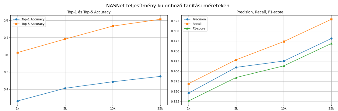
3.138. ábra. Összehasonlító metrika grafikon a NASNet iteratív tanításáról.
