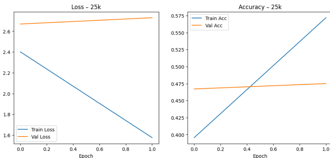
3.136. ábra. 25k adathalmazon történő tanítás grafikonja NASNet modellen.
