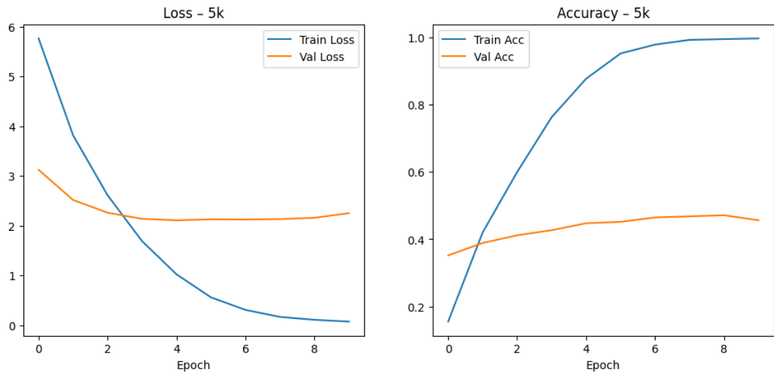
3.125. ábra. 5k adathalmazon történő tanítás grafikonja Inception-v3 modellen.
