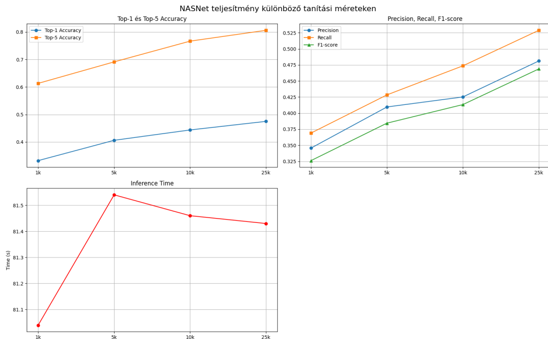
3.142. ábra. Összehasonlító grafikon a NASNet iteratív tanításáról.
