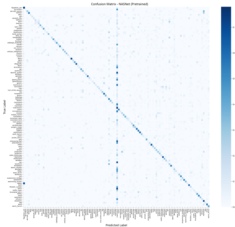
3.14. ábra. NASNet@ImageNet1k tanítás nélküli normalizált Confusion Mátrix
