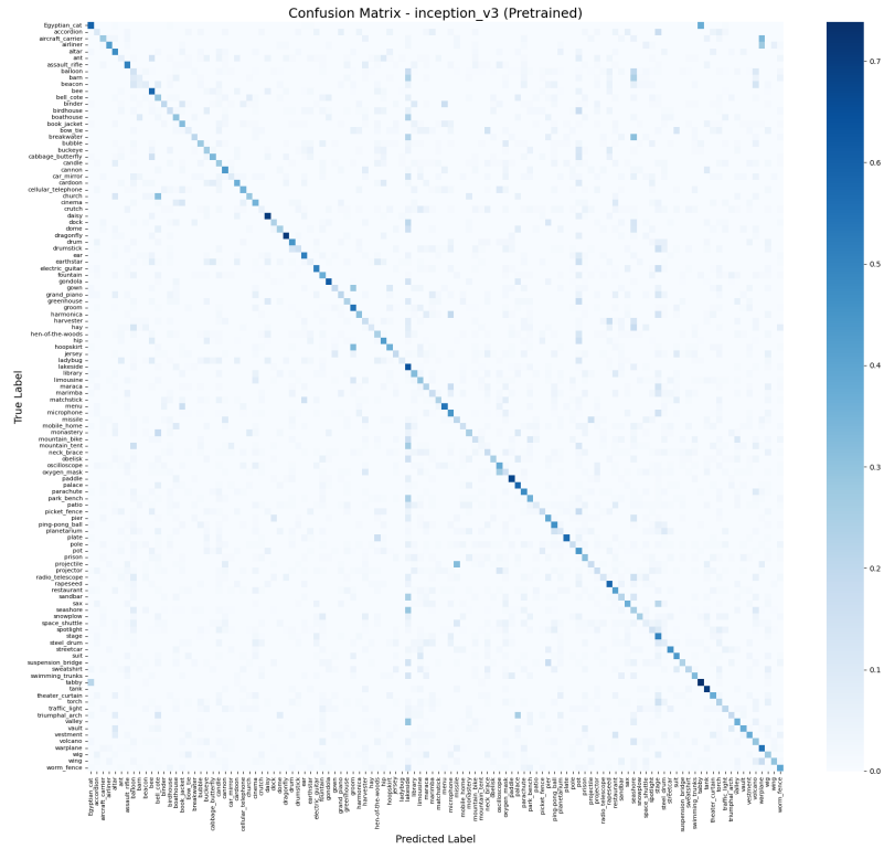
3.12. ábra. Inception-v3@ImageNet1k tanítás nélküli normalizált Confusion Mátrix
