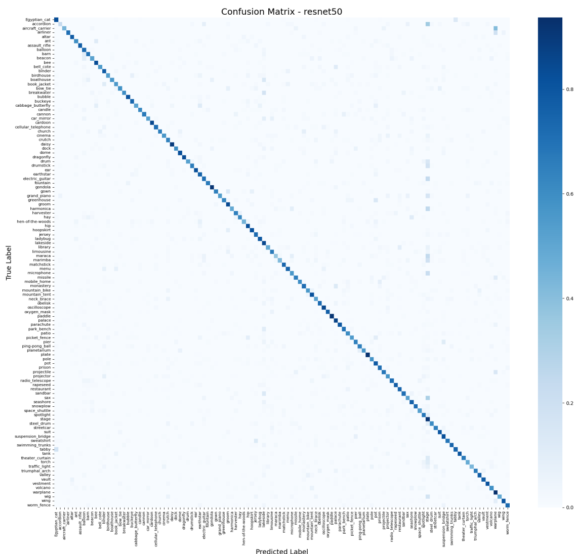
3.20. ábra. ResNet50 teljes tanítás utáni normalizált Confusion Mátrix
