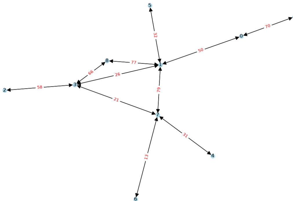
Rysunek 2.5: Przykład grafu rzadkiego analizowanego w pracy
