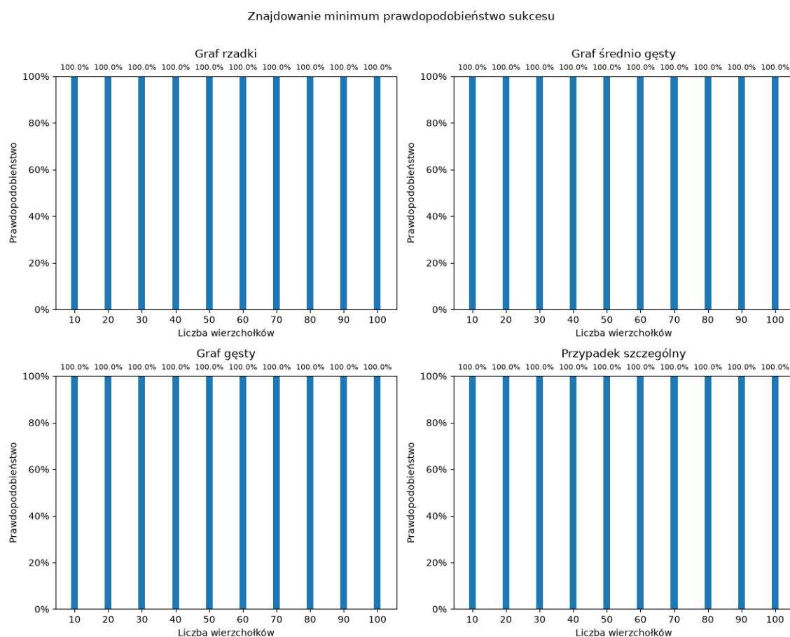
Rysunek 5.4: Prawdopodobieństwo poprawnego znalezienia minimum przez algorytm Dürre-Høyer bez limitu liczby operacji.
