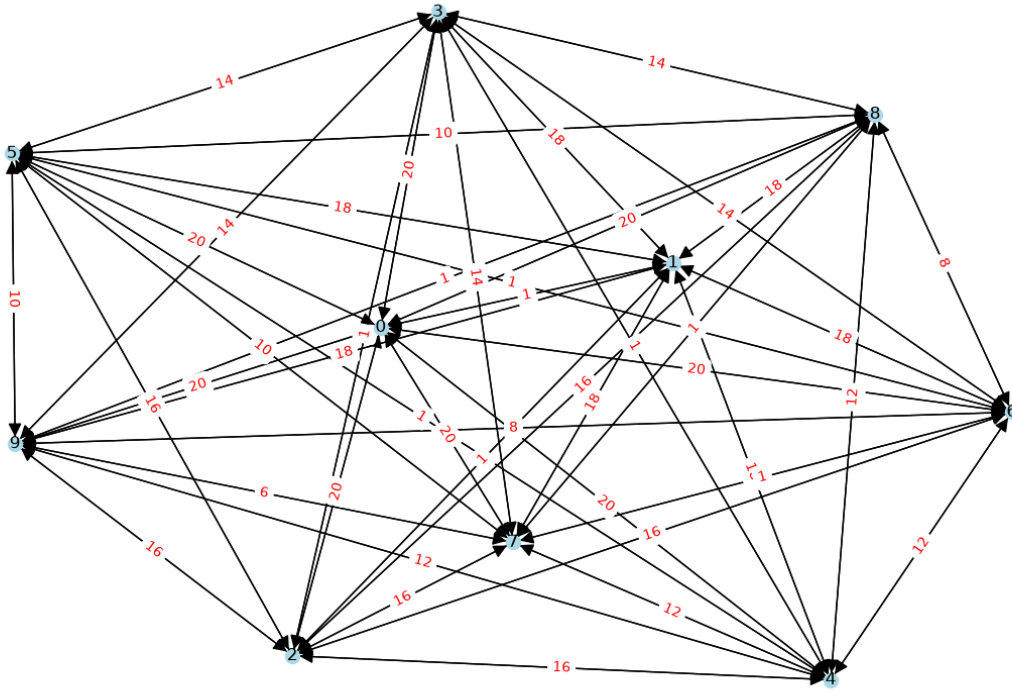
Rysunek 4.5: Przykład przypadku szczególnego dla 10 wierzchołków.
