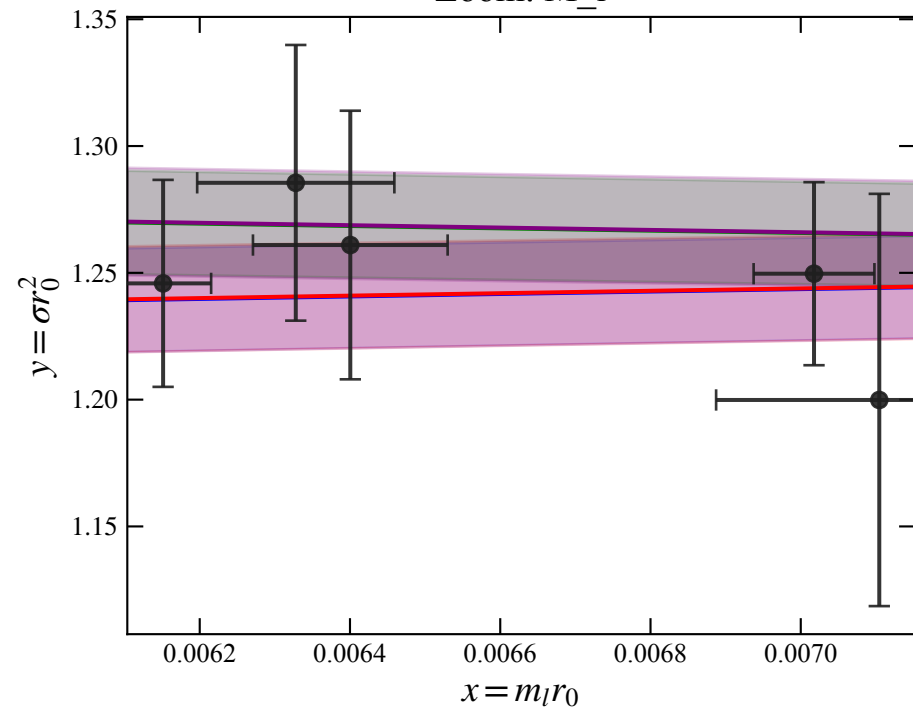
Zoom: M_i
