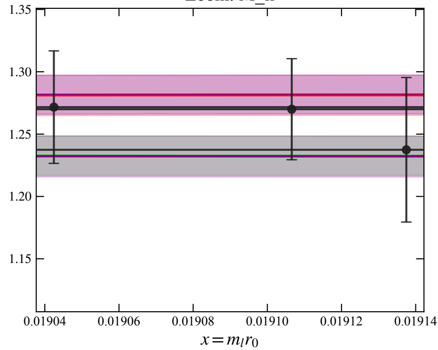
Zoom: M_ii
