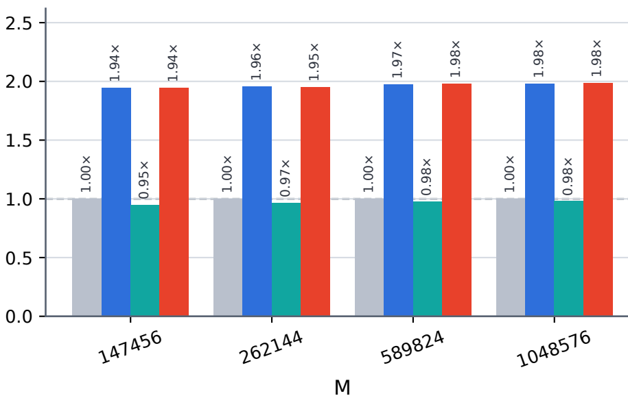
d = 768
