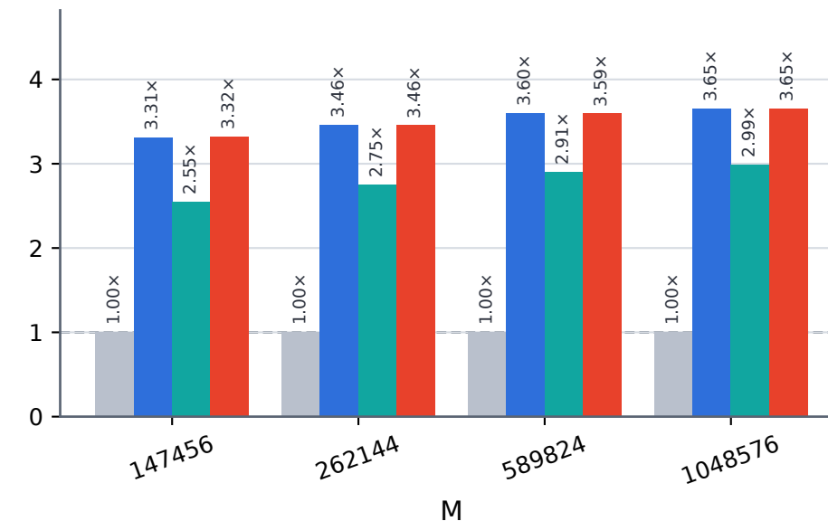
d = 768
