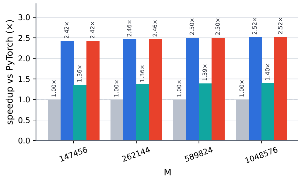
d = 512
