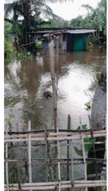
Naduar RC, Sonitpur
